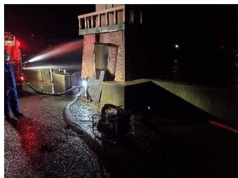
王子前ポンプ場 排水作業
