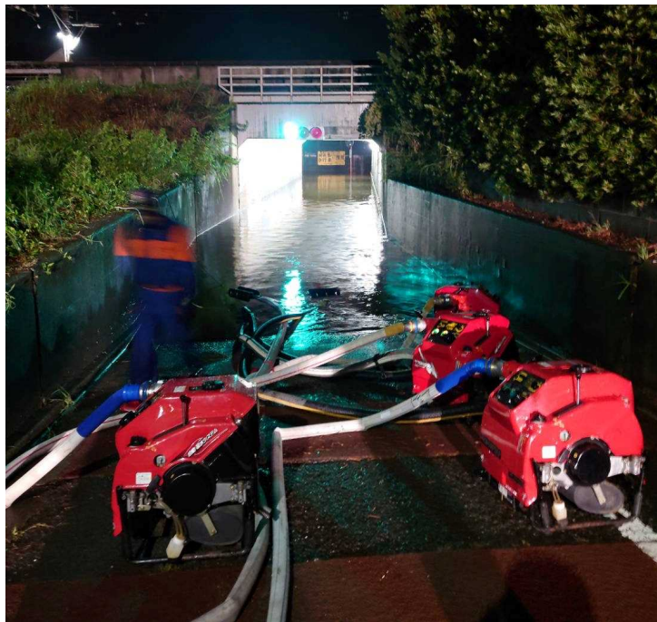
可搬ポンプによる排水作業 (一宮町一宮9275-2番地先)
