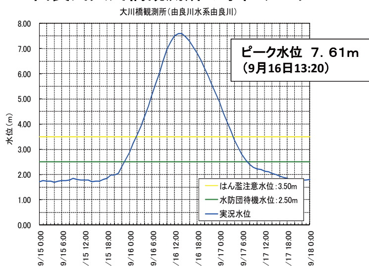
由良川大川橋観測所の水位データ
