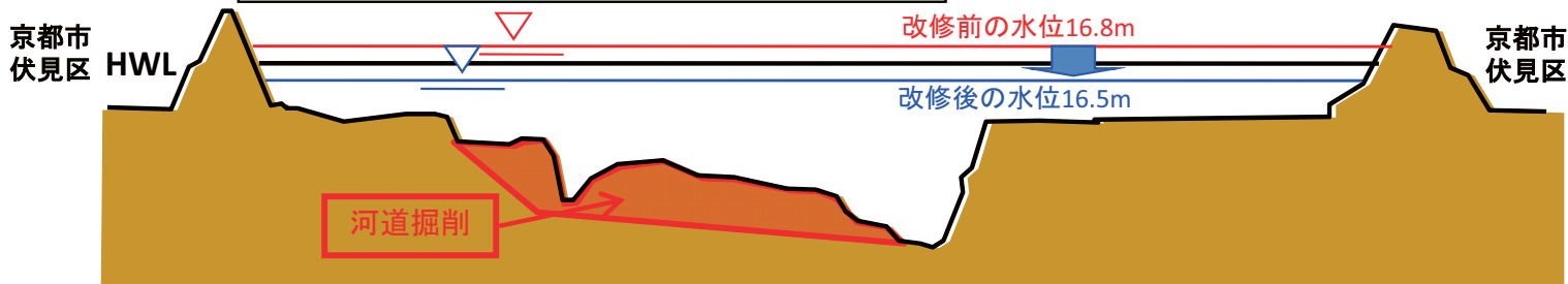
掘削済区間(1.6k地点)での水位低下効果(精査中)
