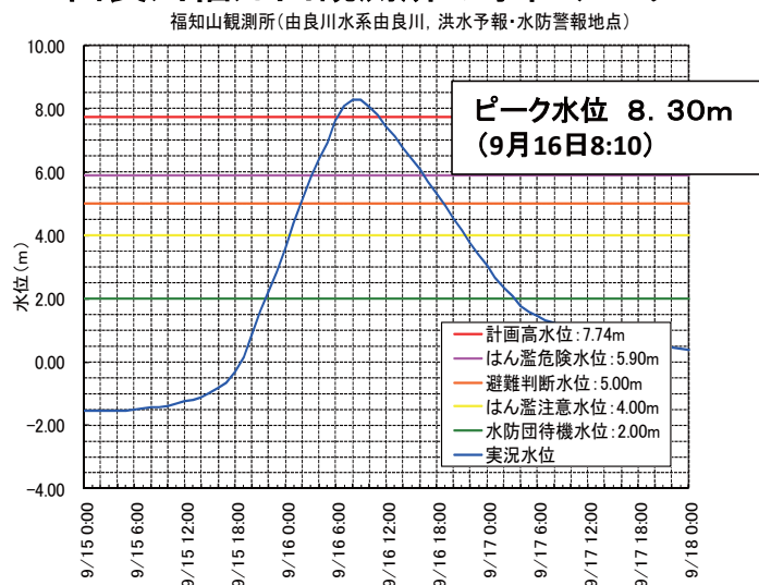
由良川福知山観測所の水位データ
