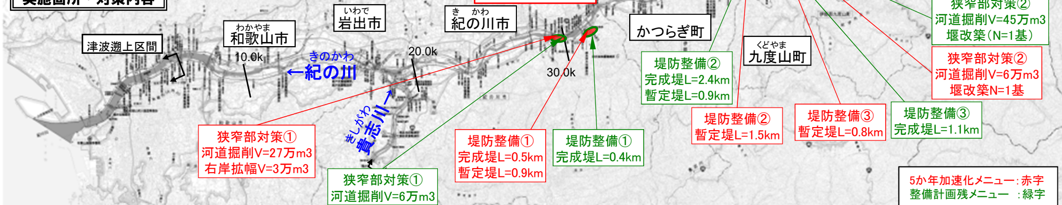
堤防整備①麻生津地区、狭窄部対策①藤崎地区
