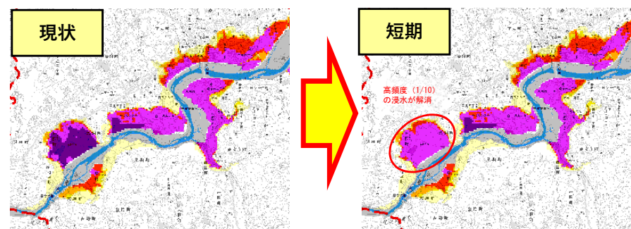
堤防整備④上野地区、堤防整備⑤二見地区
