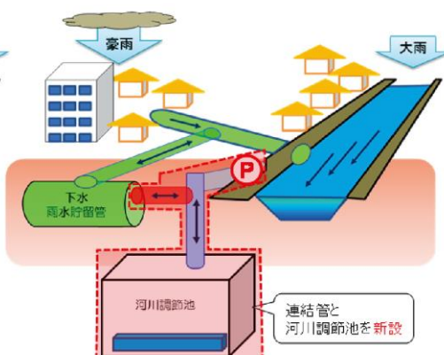
連結管及び河川調節池等を新設する場合
