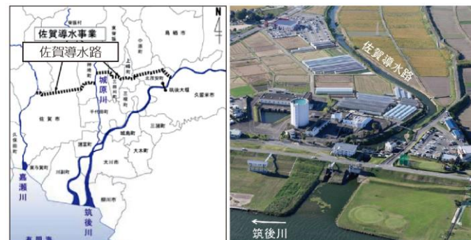
さが 佐賀導水路（佐賀県）
