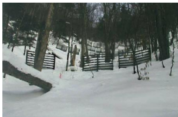
● 雪崩予防柵工(長野県松本市安曇)
