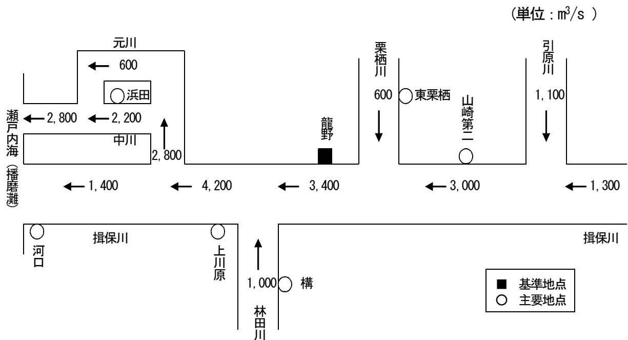
揖保川計画高水流量図
