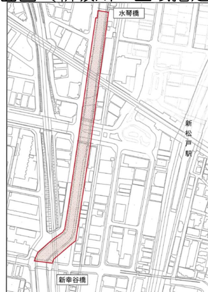
平面図（新坂川 区域指定）
