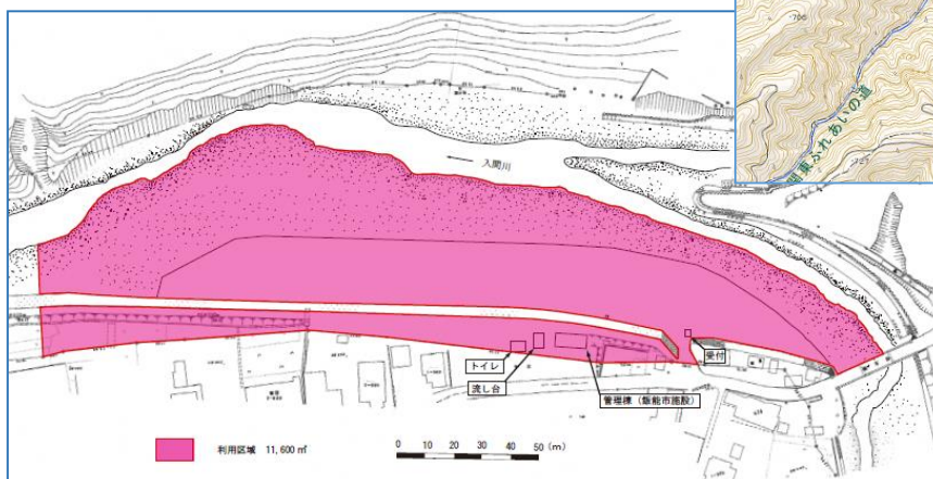
平面図（名栗弁天河原河川広場）
