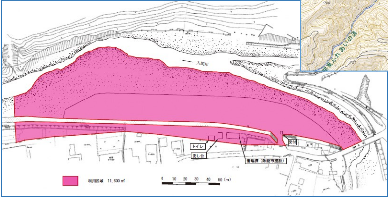
平面図（名栗弁天河原河川広場）
