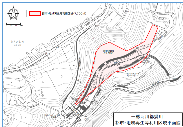
平面図（ときがわ町木のむらキャンプ場）
