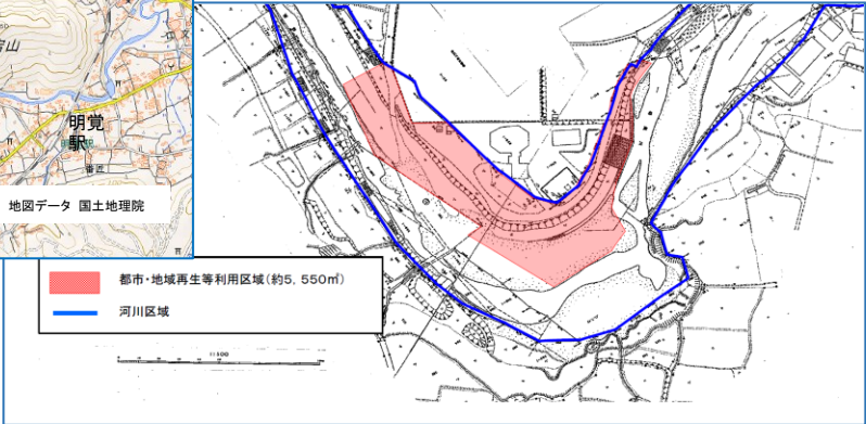
平面図（都幾川河川敷）
