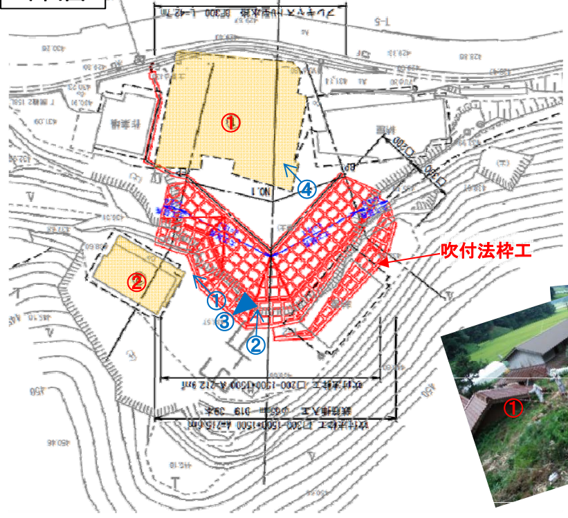
平面図
