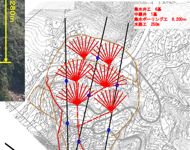
対策工平面図
