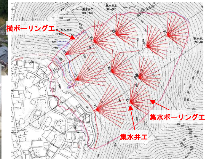
対策工平面図
