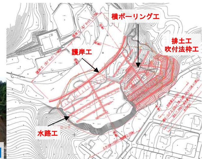
対策工平面図
