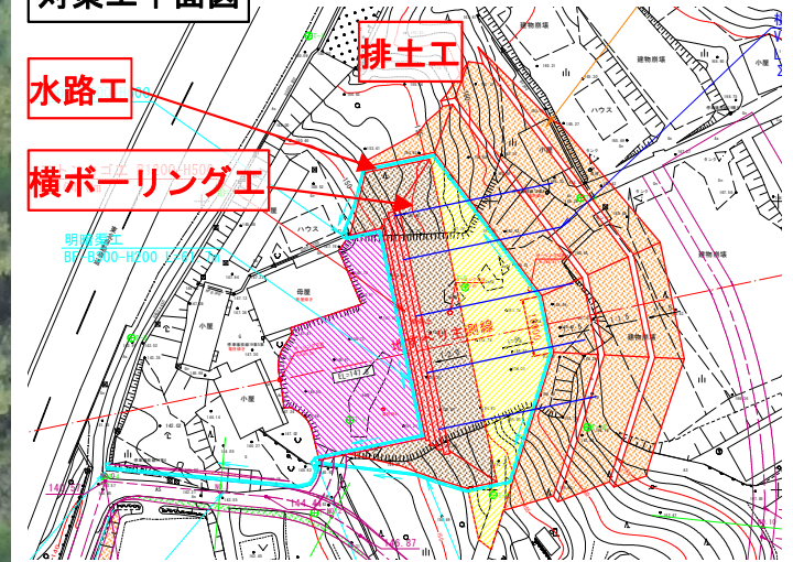
対策工平面図
