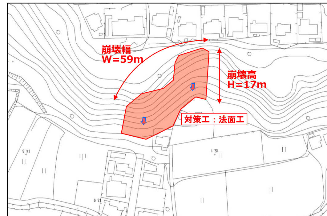
斜面崩壊状況
