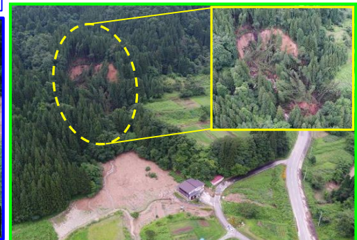
地すべり
