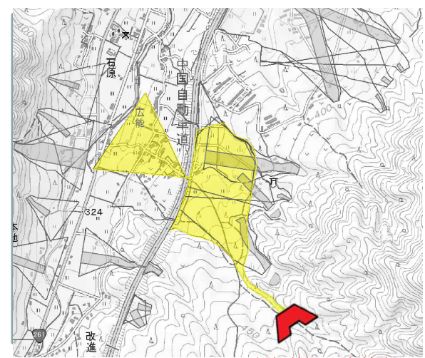
土砂を捕捉した砂防堰堤 警戒区域内の保全家屋16戸
