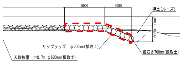
横断面図
