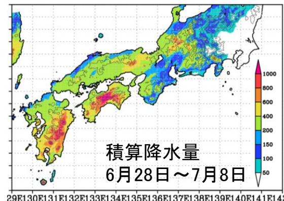
通常のJRA-55からの 再現実験
