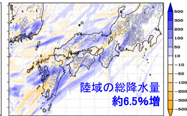
再現実験と近年の気温上昇を 引いた感度実験との差
