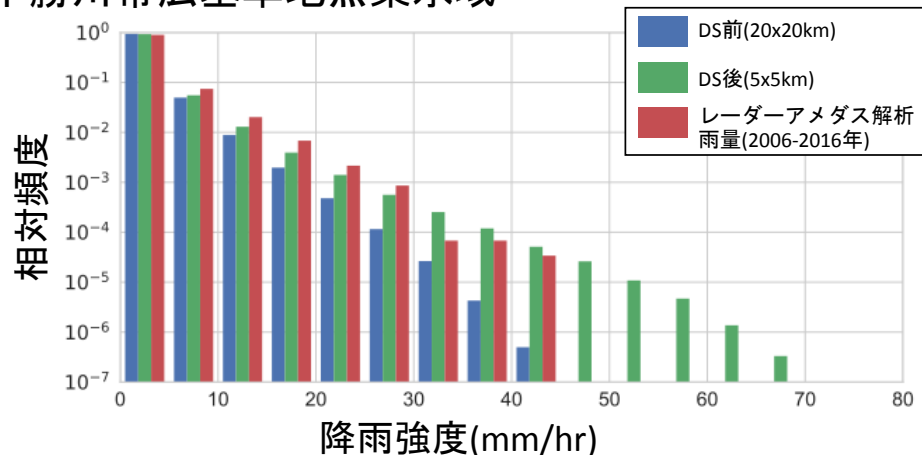
十勝川帯広基準地点集水域
