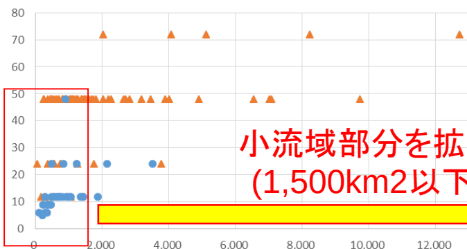
地点上流面積－降雨継続時間
