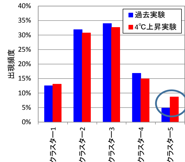
クラスター毎の出現頻度の比較
