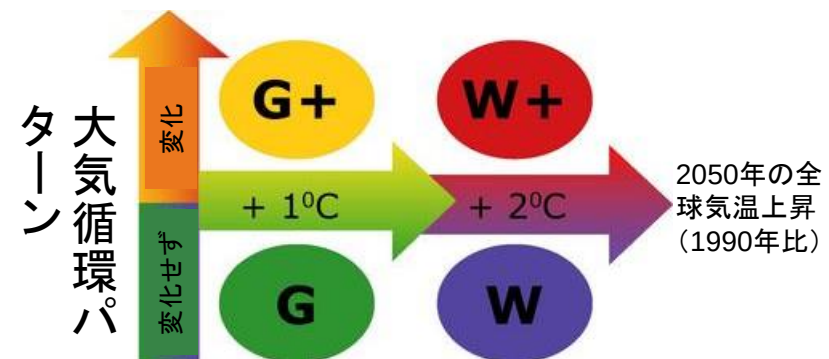
図2 KNMI'06の4シナリオ※5
