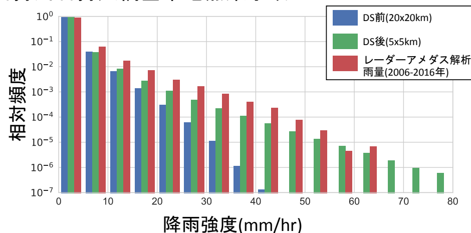
石狩川石狩大橋基準地点集水域
