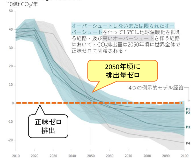
世界全体のCO 2 正味排出量
