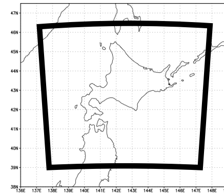
計算領域1(北海道)
