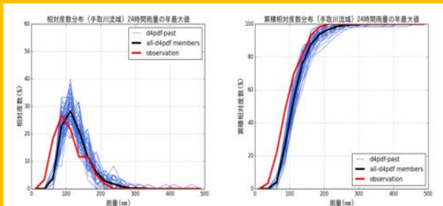
手取川(再現性が低い例)
