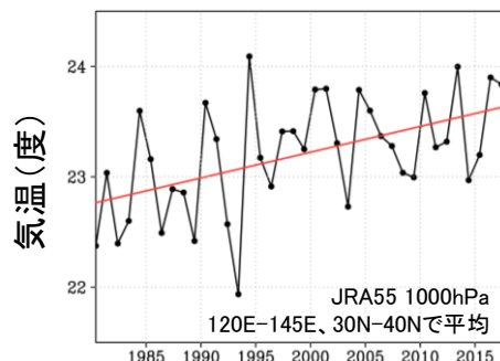
夏季(JJA)平均気温の時系列と線形トレンド 1980-2018年(西日本)
