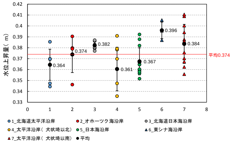
海面水位の上昇量の予測結果
