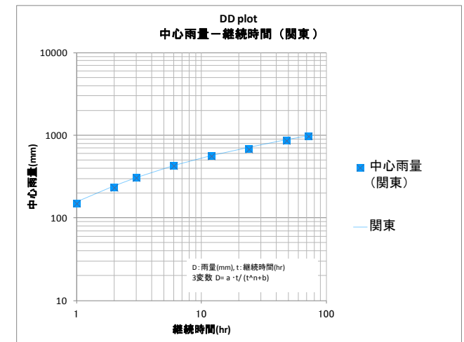
関東地区のDD図
