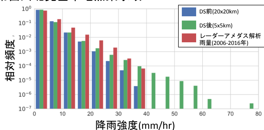
常呂川北見基準地点集水域
