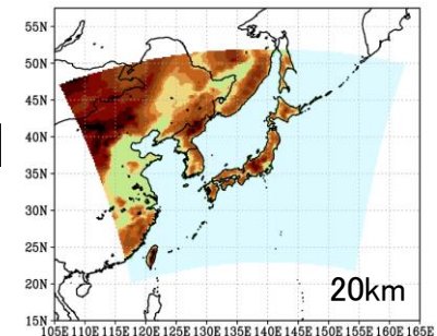
JRA-55を境界値として 20km=>5km=>2kmの ダウンスケーリングby NHRGM
