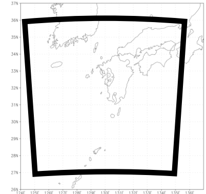
計算領域2(中国, 四国, 九州)
