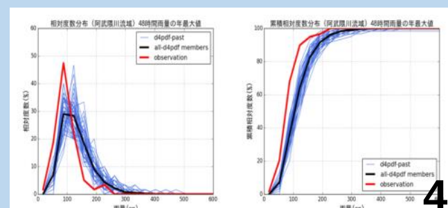
阿武隈川(再現性が低い例)
