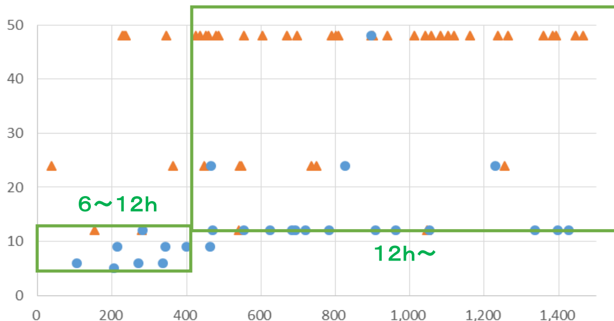
地点上流面積－降雨継続時間
