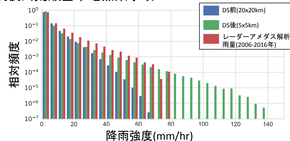
筑後川荒瀬基準地点集水域
