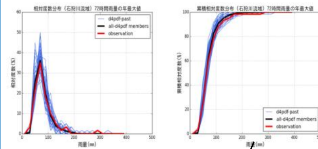
石狩川(再現性が高い例)
