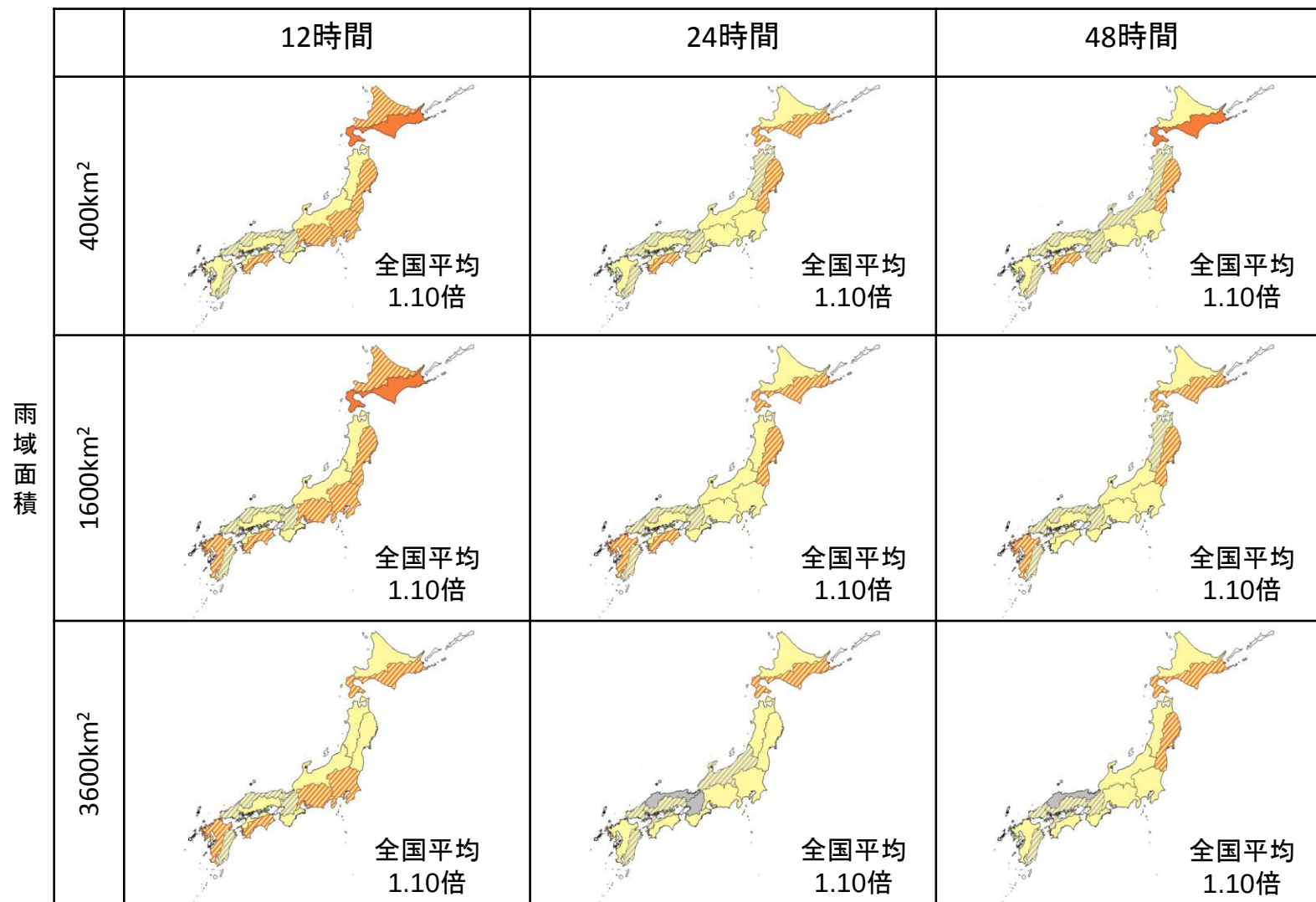
降雨継続時間
