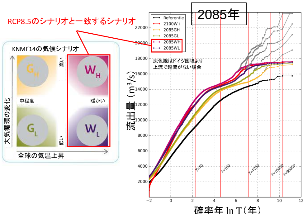
ライン川の流量確率の将来予測 ※1
