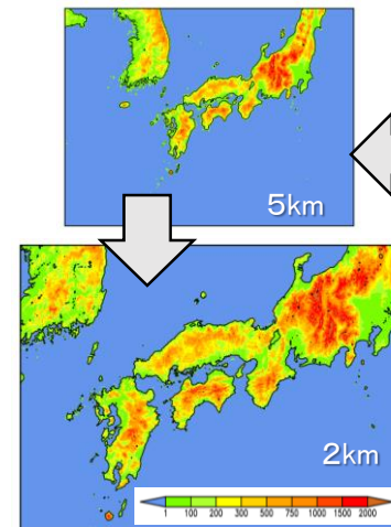
通常のJRA-55からの 再現実験
