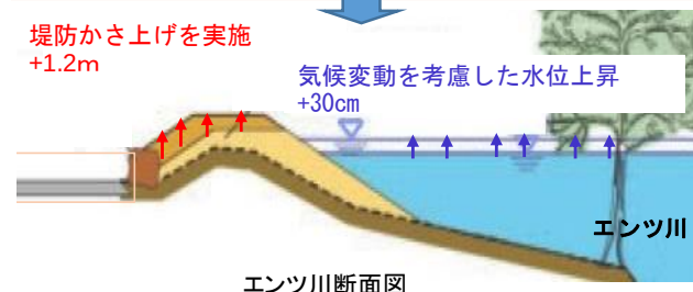
エンツ川断面図
