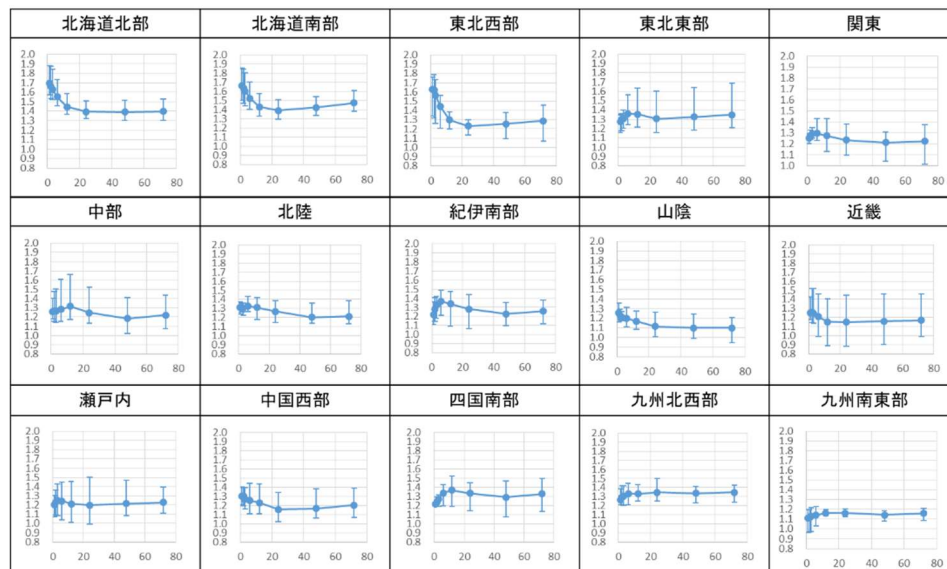
図-17 地域区分毎の降雨継続時間と降雨量変化倍率の関係性
