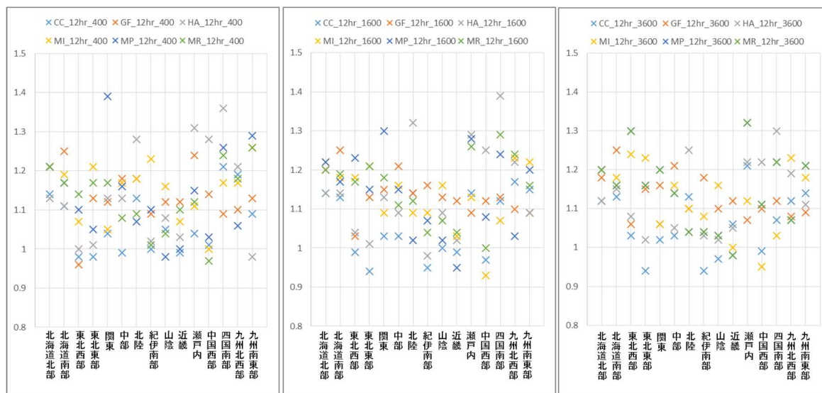
図-18 各地域区分における降雨継続時間 12 時間の海面水温モデル毎の降雨量変化倍率 (左から雨域面積 400km 2 、1600km 2 、3600km 2 )
