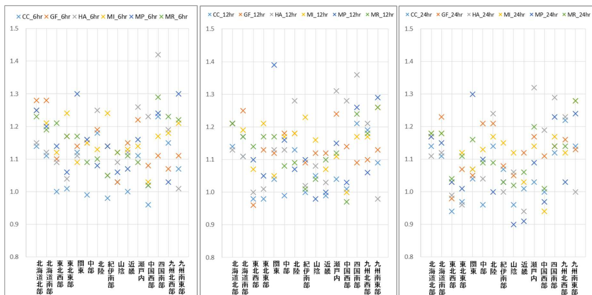
図-24 各地域区分における雨域面積 400km 2 の海面水温モデル毎の降雨量変化倍率 (左から降雨継続時間 6 時間、12 時間、24 時間) ※降雨継続時間 12 時間、24 時間は再掲
