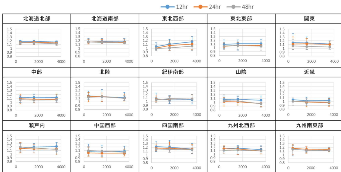
図-21 地域区分毎の雨域面積と降雨量変化倍率の関係性 (降雨継続時間 12 時間を青線、24 時間を橙線、48 時間を灰線で表している)
