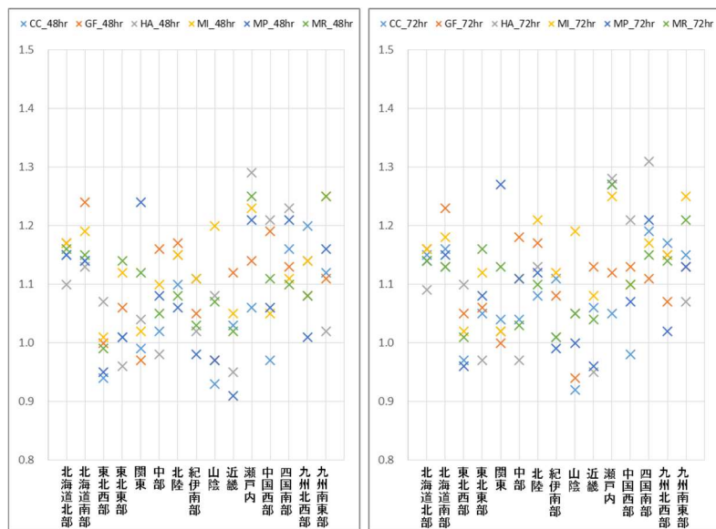
図-25 各地域区分における雨域面積 400km 2 の海面水温モデル毎の降雨量変化倍率 (左から降雨継続時間 48 時間、72 時間) ※降雨継続時間 48 時間は再掲
