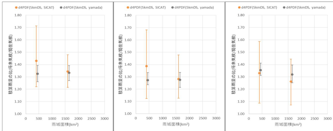
図-27 筑後川流域における d4PDF (5km, SI-CAT)、 d4PDF (5km, yamada) を用いた降雨量変化倍率の比較 (左から降雨継続時間 12 時間、24 時間、48 時間)
