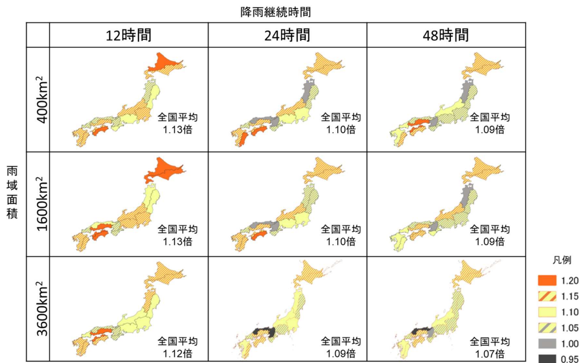
図-22 各地域区分の海面水温 6 パターンによる降雨量変化倍率の平均値
