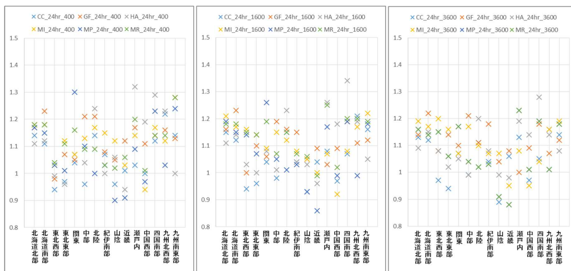
図-19 各地域区分における降雨継続時間 24 時間の海面水温モデル毎の降雨量変化倍率 (左から雨域面積 400km 2 、1600km 2 、3600km 2 )
