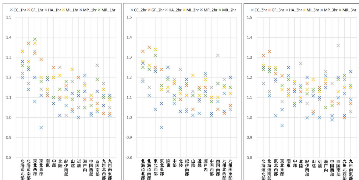
図-23 各地域区分における雨域面積 400km 2 の海面水温モデル毎の降雨量変化倍率 (左から降雨継続時間 1 時間、2 時間、3 時間)
