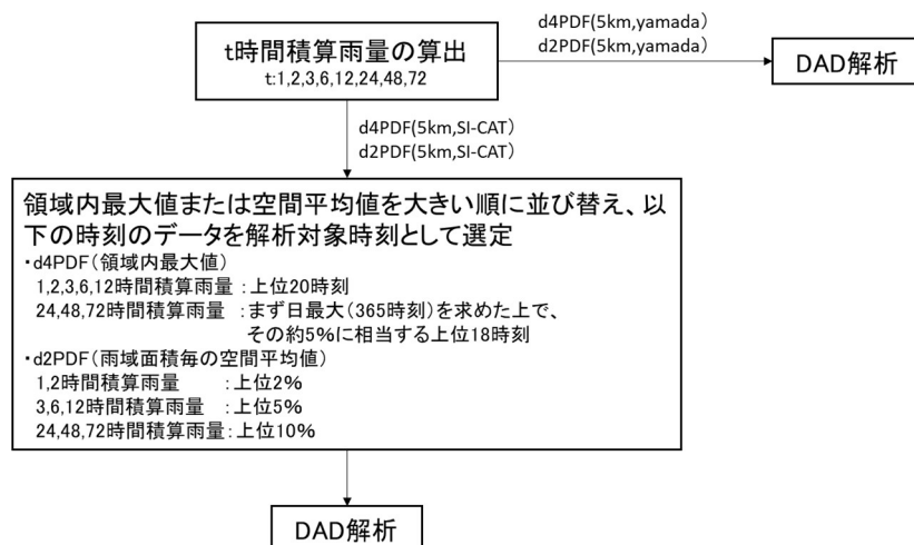
図-4 DAD 解析対象時刻の選定フロー
