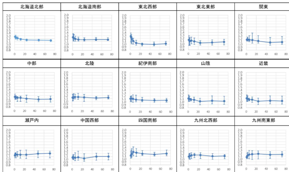
図-26 地域区分毎の降雨継続時間と降雨量変化倍率の関係性
