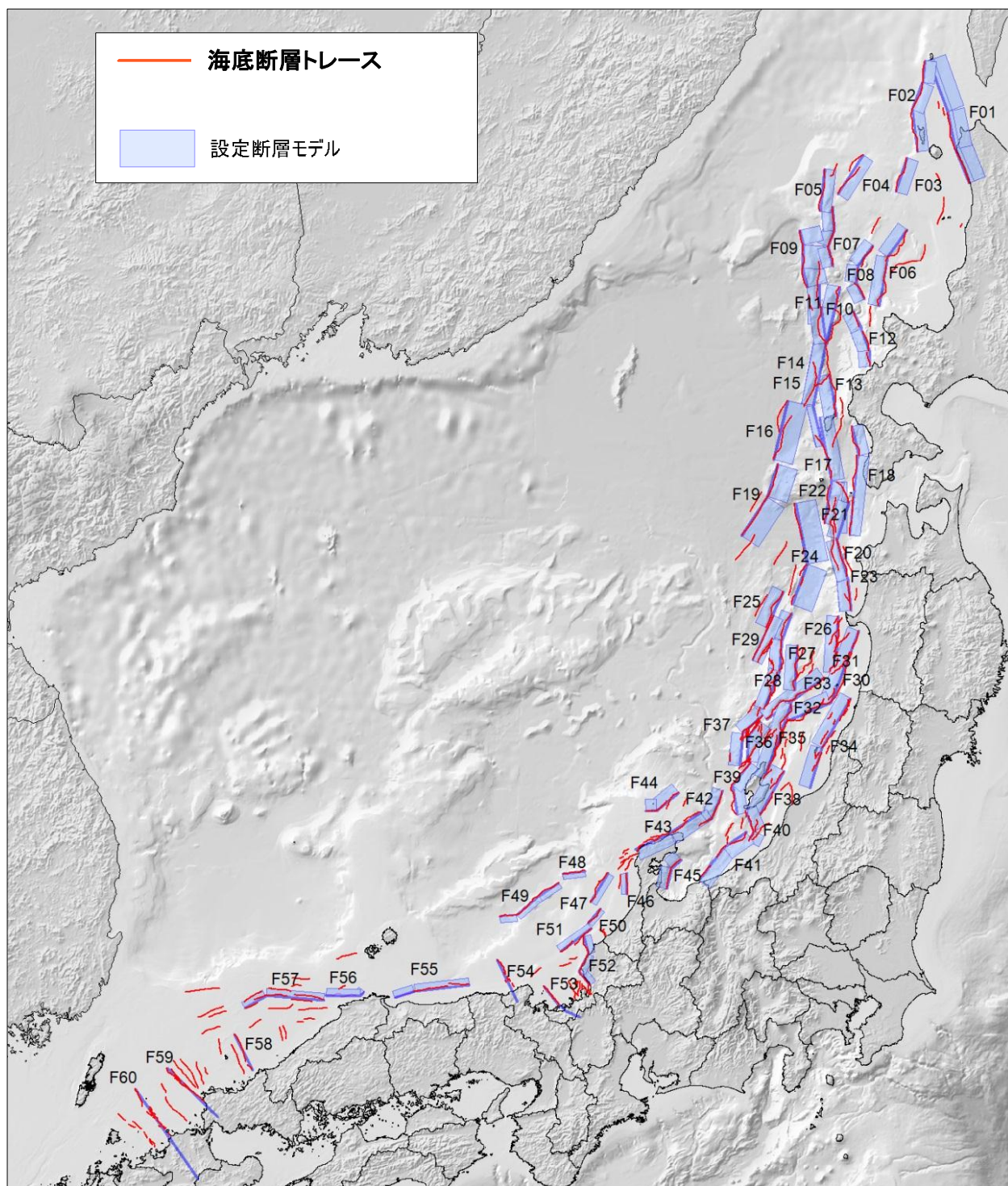
図50－1 今回設定した津波断層モデルの位置(全国)
