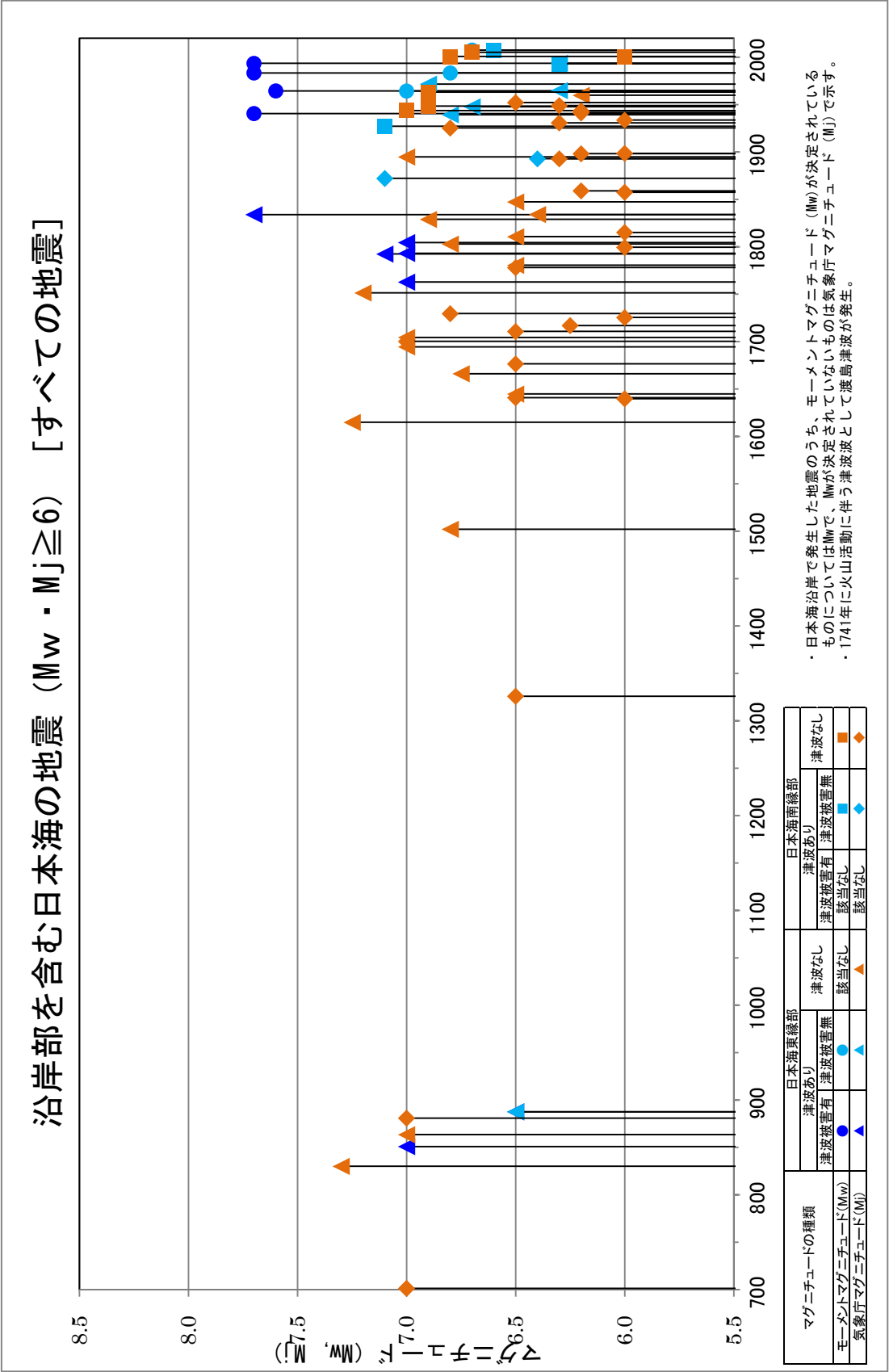
図5 沿岸部を含む日本海における地震 ( M \geq 6 ) の発生履歴 (西暦 700 年以降)
