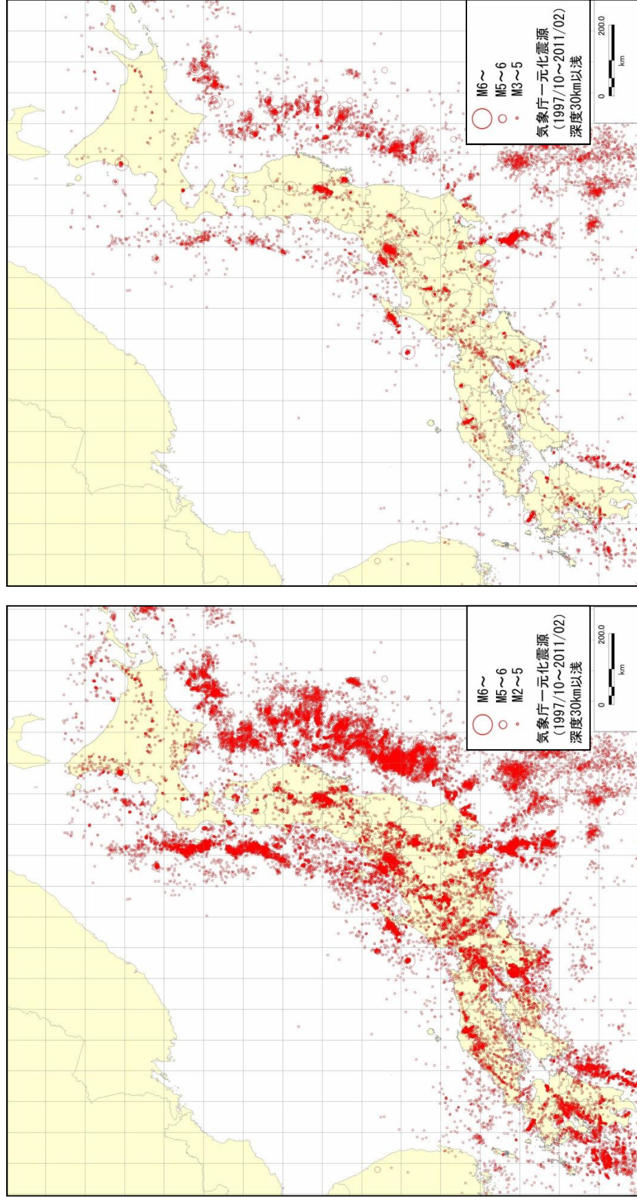
図1 日本周辺の地震活動
