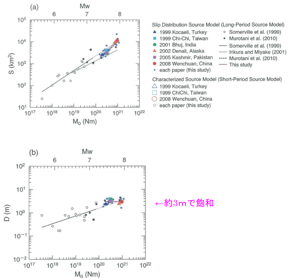
図 3 6 Murotani et al. (2010) および田島ほか (2013) のスケーリング式
