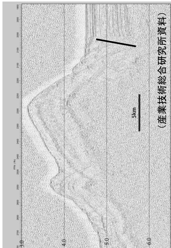
図26-2 奥尻島北方の奥尻海嶺
