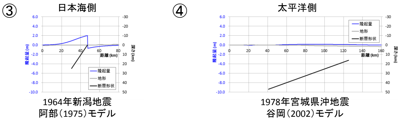
図59-4 同程度の地震規模の地震による海底面の地殻変動の比較
