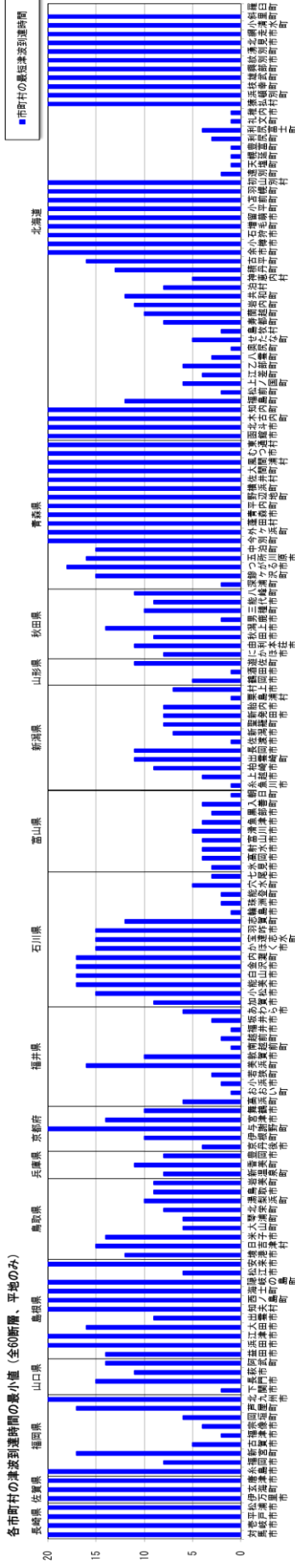
図60 60断層モデルの津波到達時間の最小値
