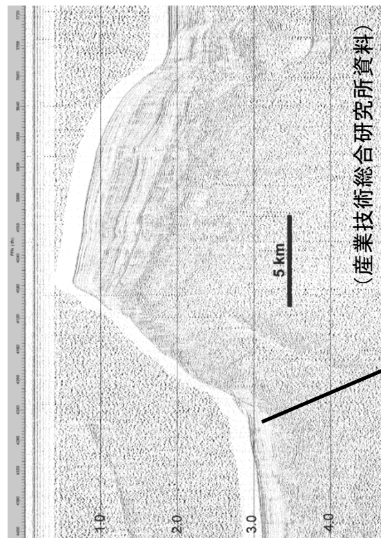
図26-3 奥尻島南方の奥尻海嶺
