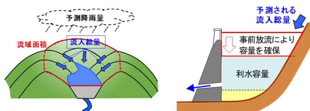
図表 4-4 事前放流の開始基準と水位低下量の設定方法（簡易な手法）
