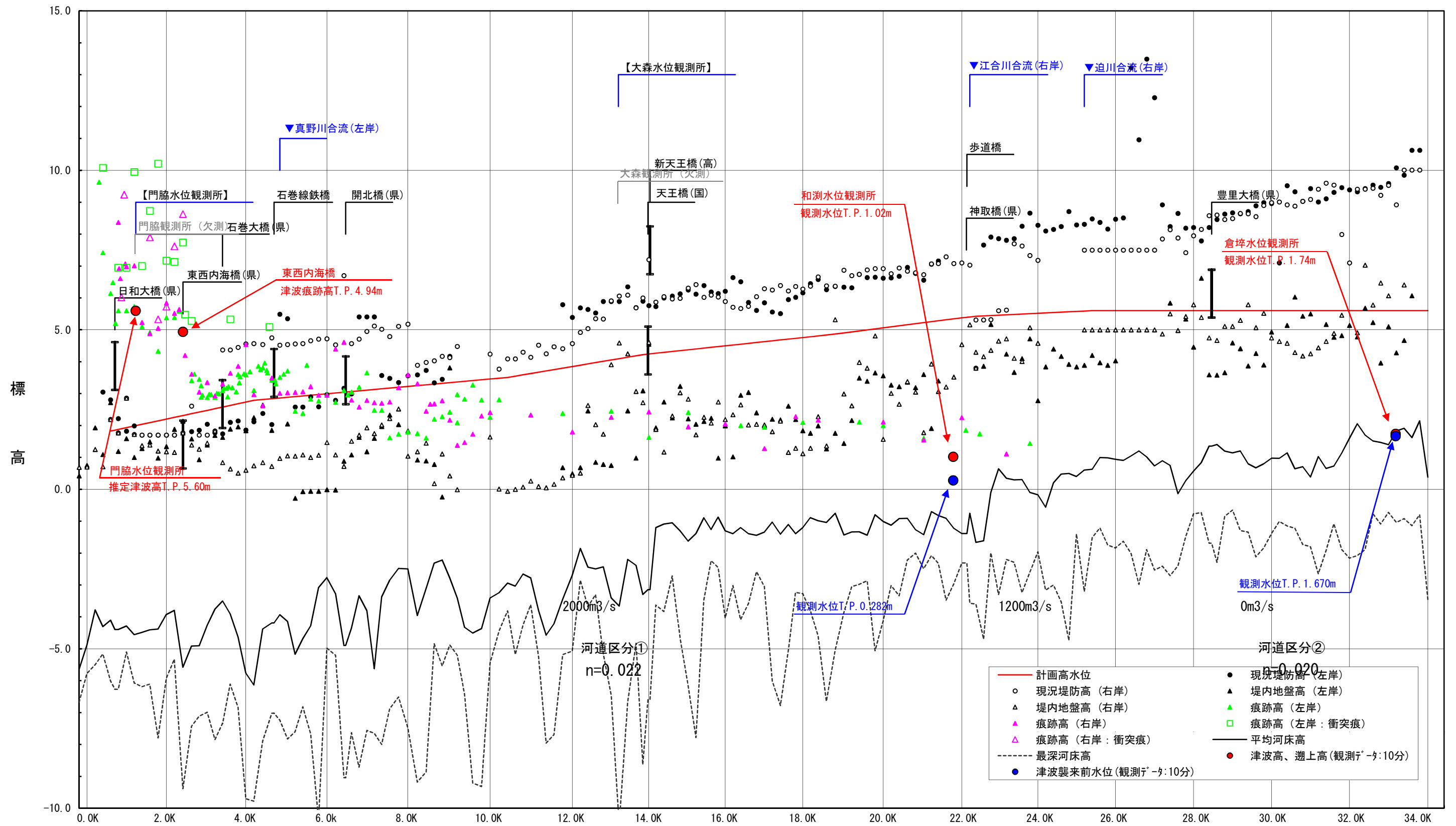
旧北上川：整備計画河道計算水位縦断面図
