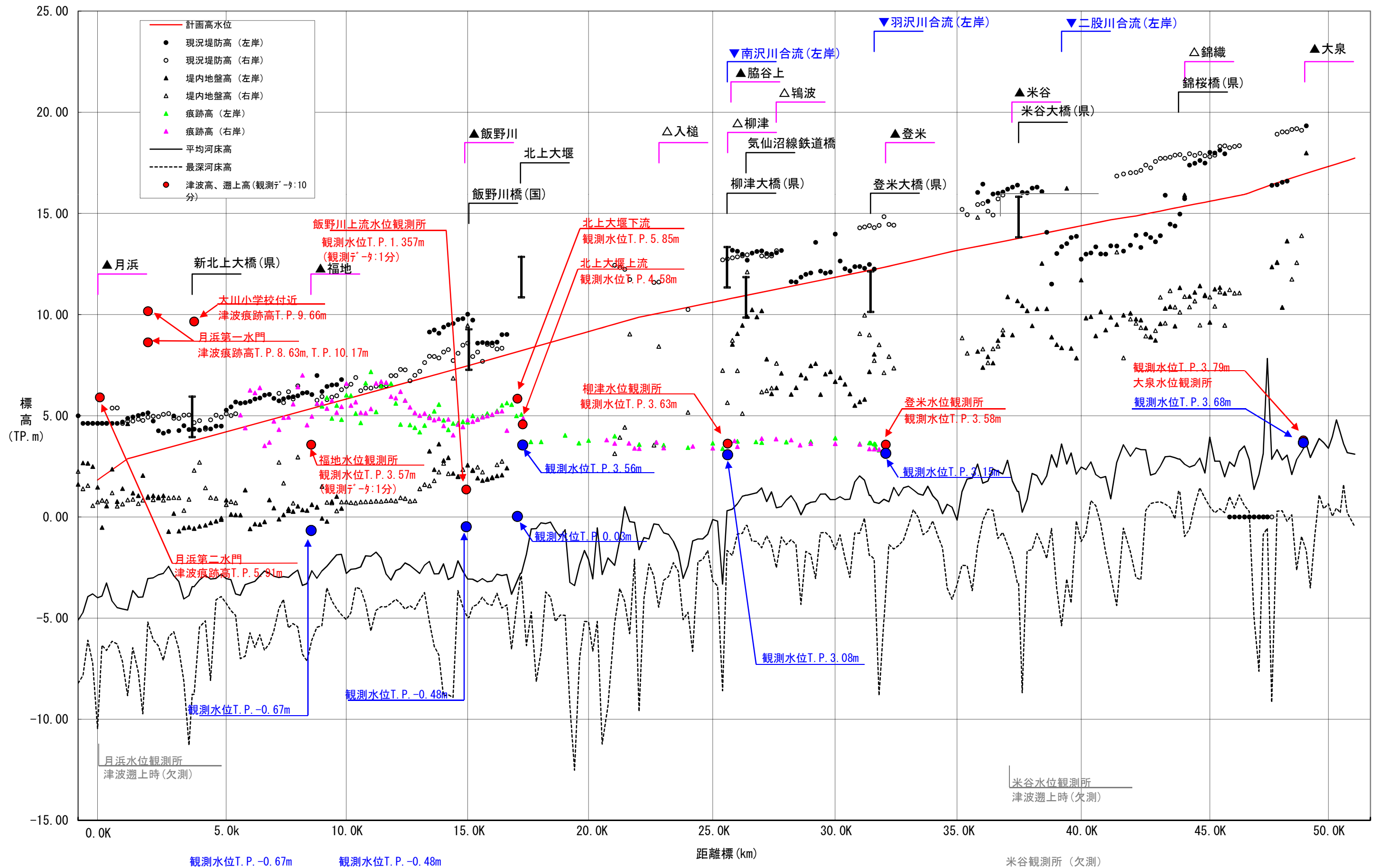
北上川〔宮城県〕：整備計画河道計算水位縦断面図
