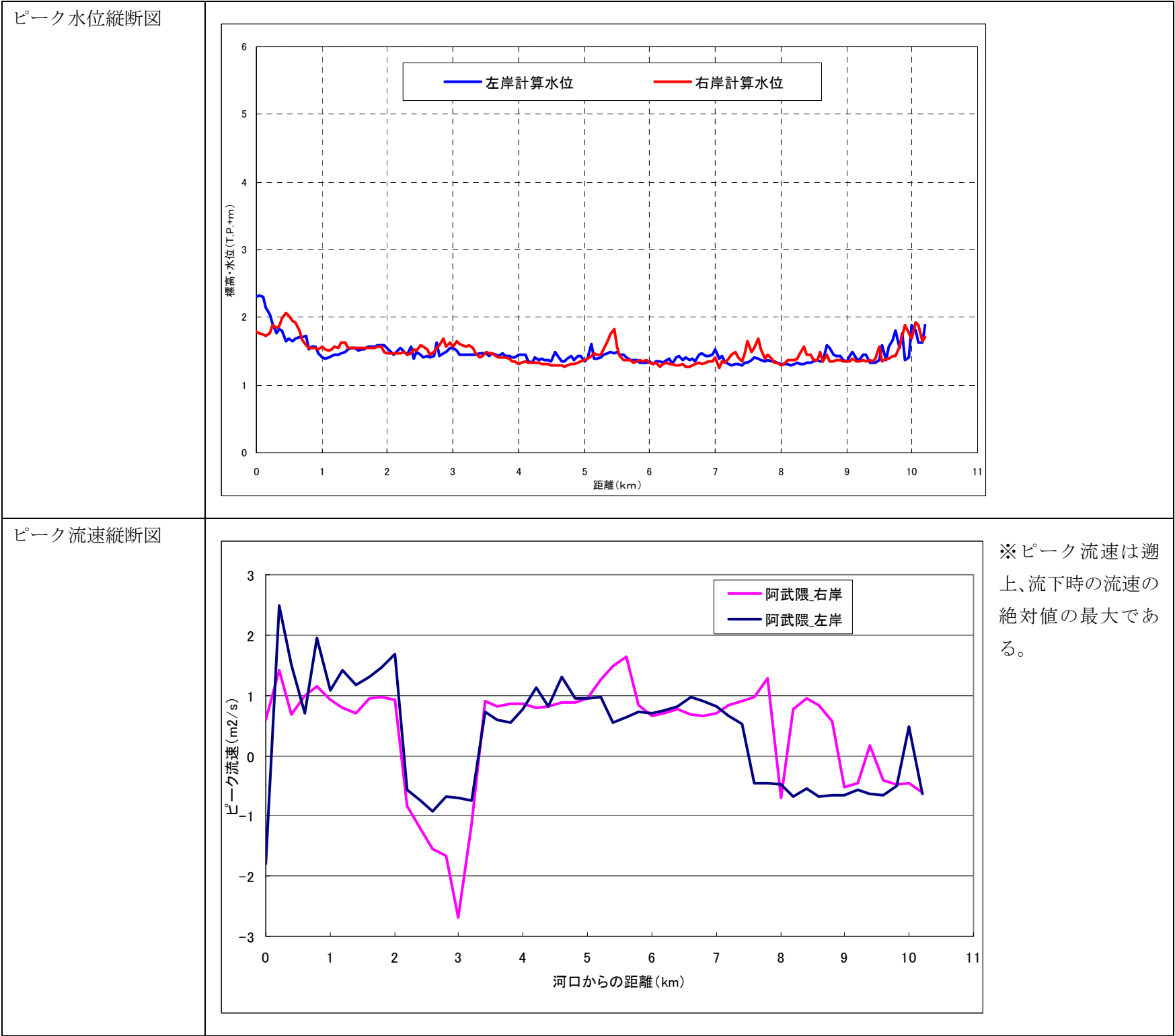
①【河道ピーク水位及び流速縦断図（想定宮城、計画河道）】 阿武隈川
