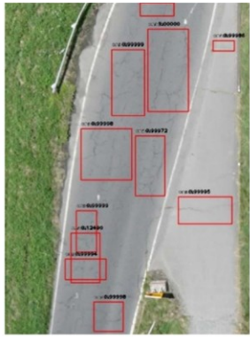
堤防天端亀裂の自動抽出 出典)令和2年度河川巡視技術検証業務その1
