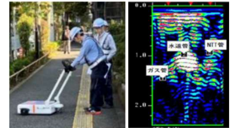
宅地開発における無電柱化実施事例
