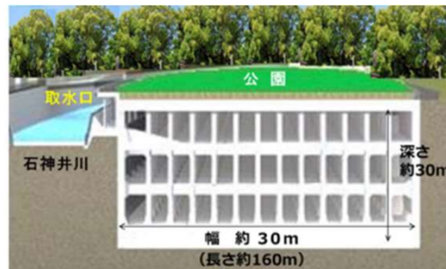
公園と連携した調節池の整備例 (城北中央公園調節池)
