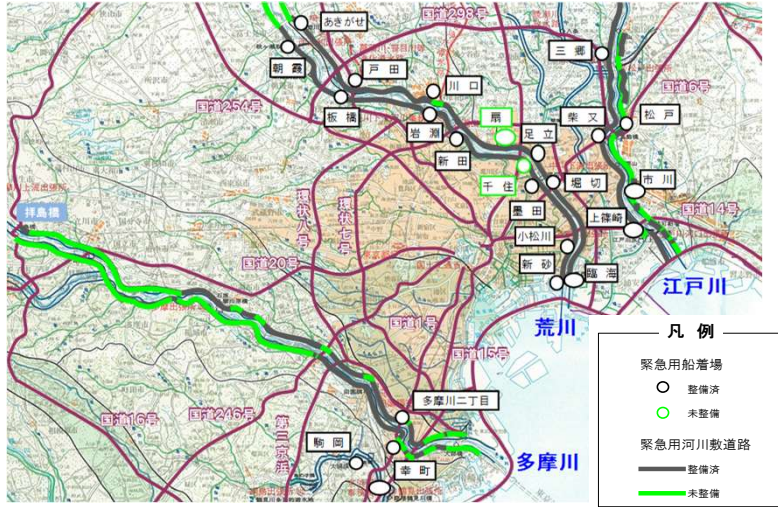
緊急用河川敷道路及び緊急用船着場 整備状況 (関東地方整備局資料)
