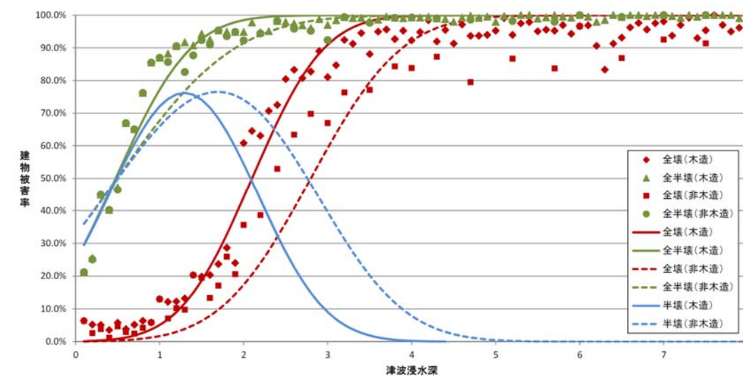
津波浸水深ごとの建物被害率(上：人口集中地区、下：人口集中地区以外)
