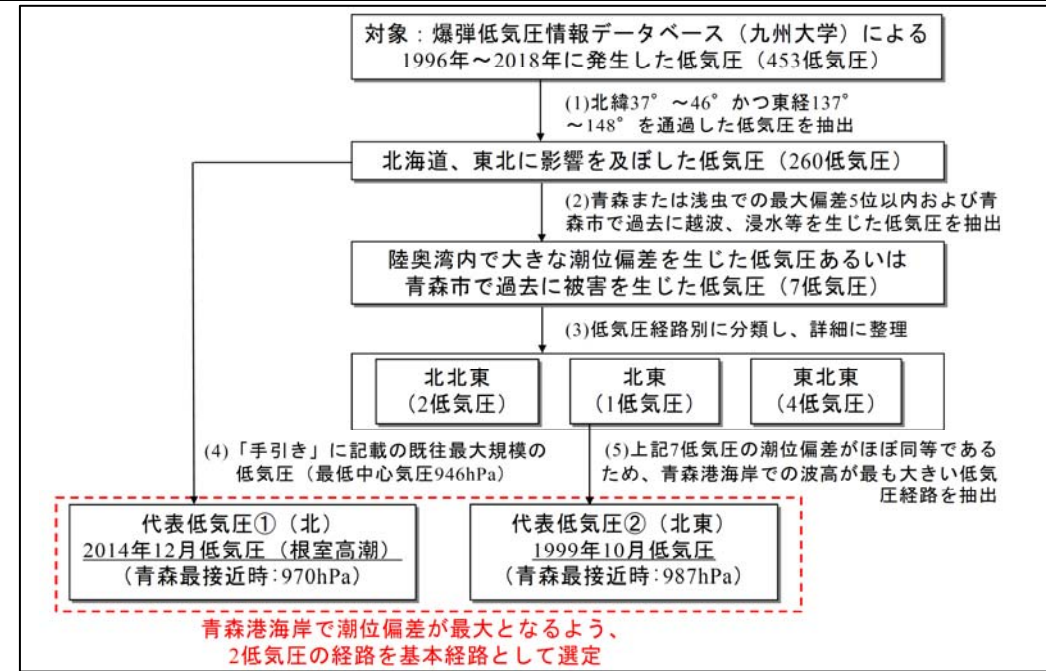
図14 低気圧事例の整理方針 9
