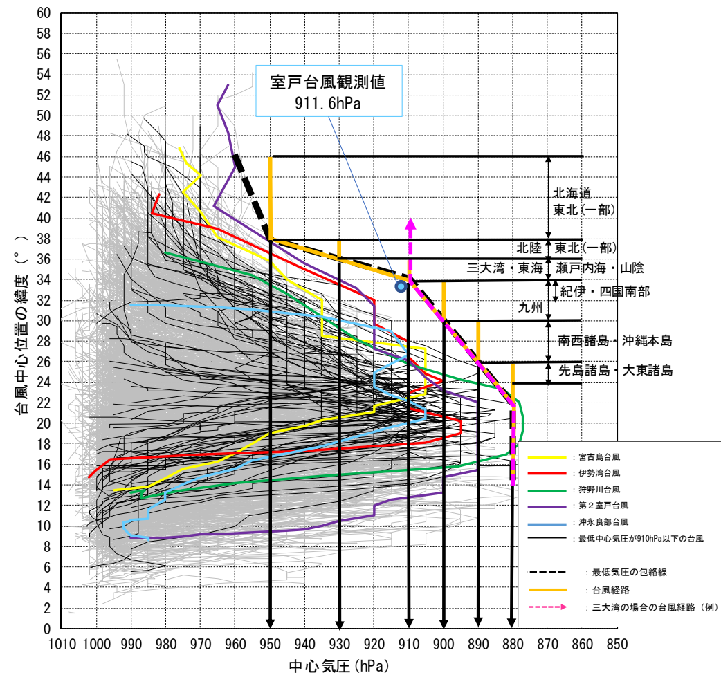
図5 想定する台風の中心気圧の設定方法
