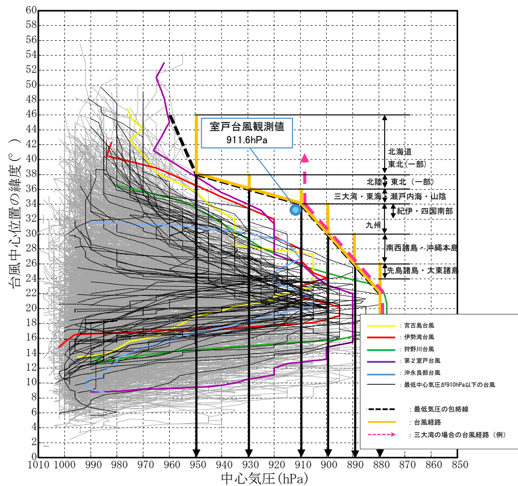
図3 想定する台風の中心気圧の設定方法
