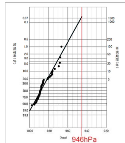
図8 2014年12月低気圧の確率評価（中心気圧） 6
