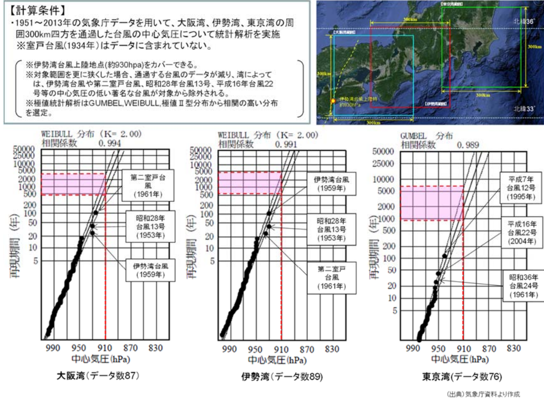
図2 1934年室戸台風の確率評価（中心気圧）
