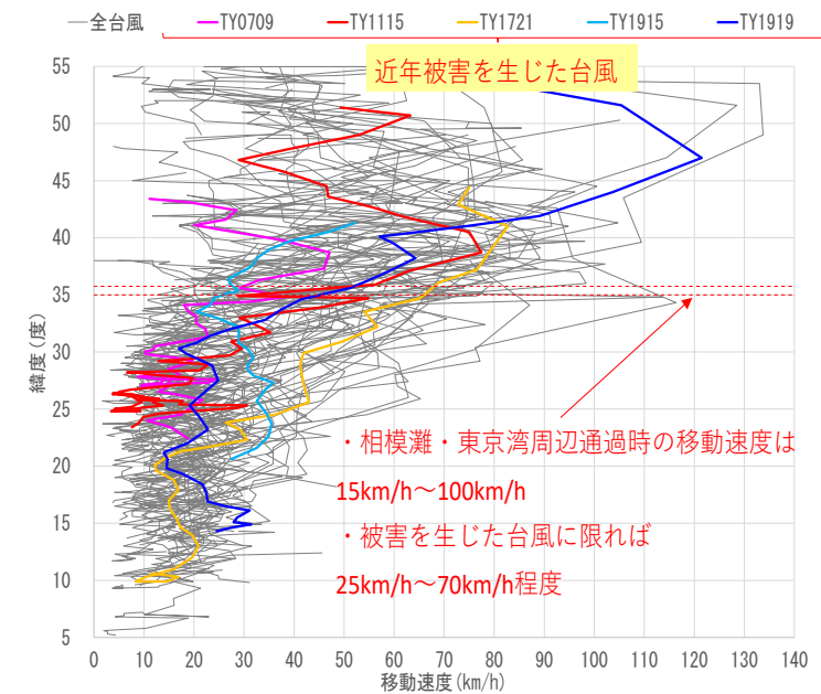
図10 相模灘・東京湾周辺を通過した台風の移動速度・緯度分布
