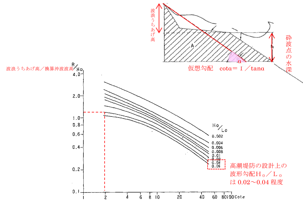
図23 改良仮想勾配法による波のうちあげ高算定図 27 （一部加筆）
