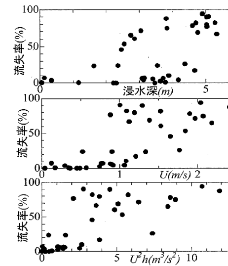
被災外力因子パラメタと家屋流失率の関係
