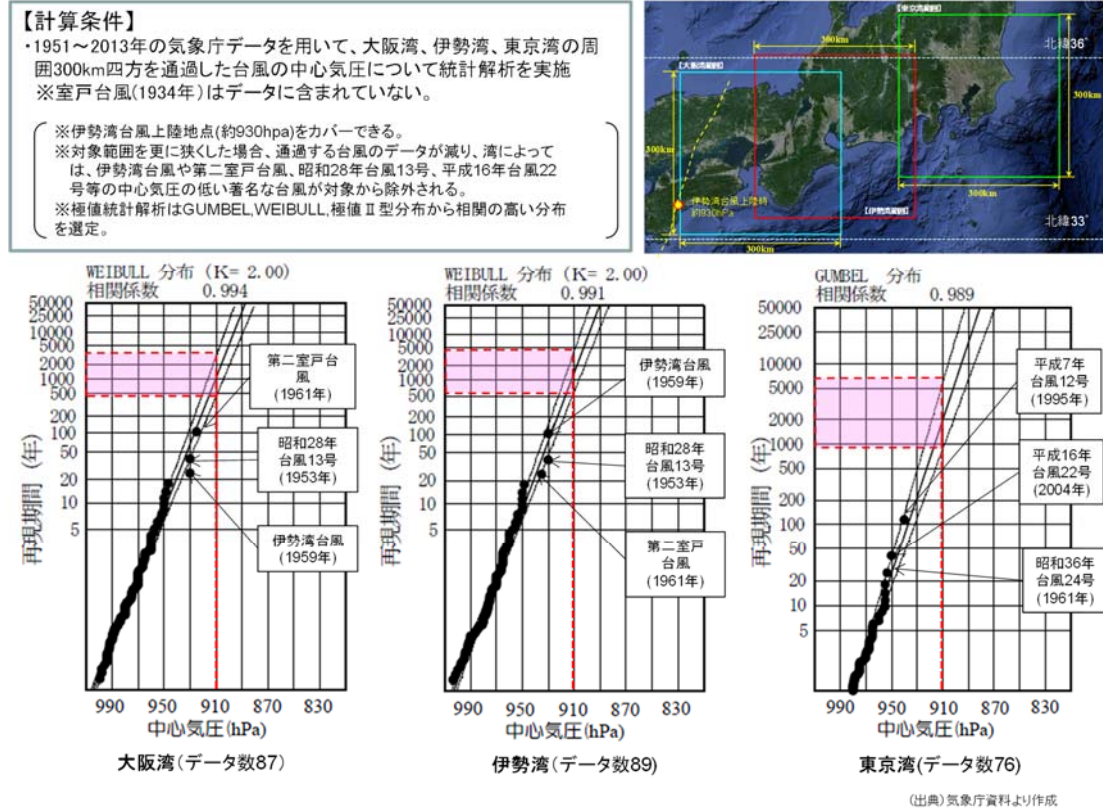
図4 1934年室戸台風の確率評価（中心気圧）
