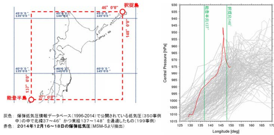
図7 2014年12月低気圧の中心気圧 5
