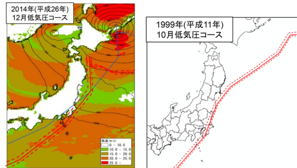
図13 想定低気圧経路図 8
