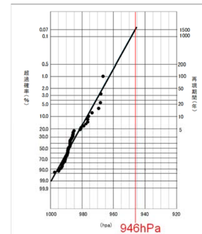
図16 2014年12月低気圧の確率評価（中心気圧） 11
