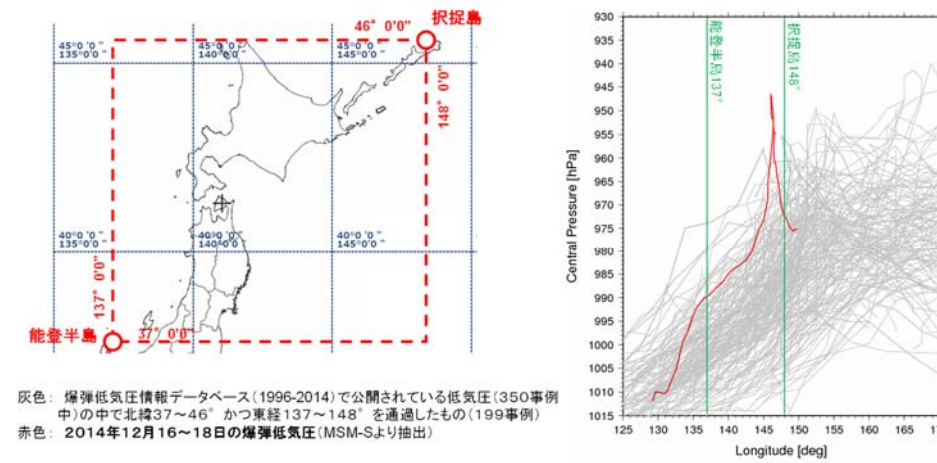
図14 低気圧事例の整理方針 9
