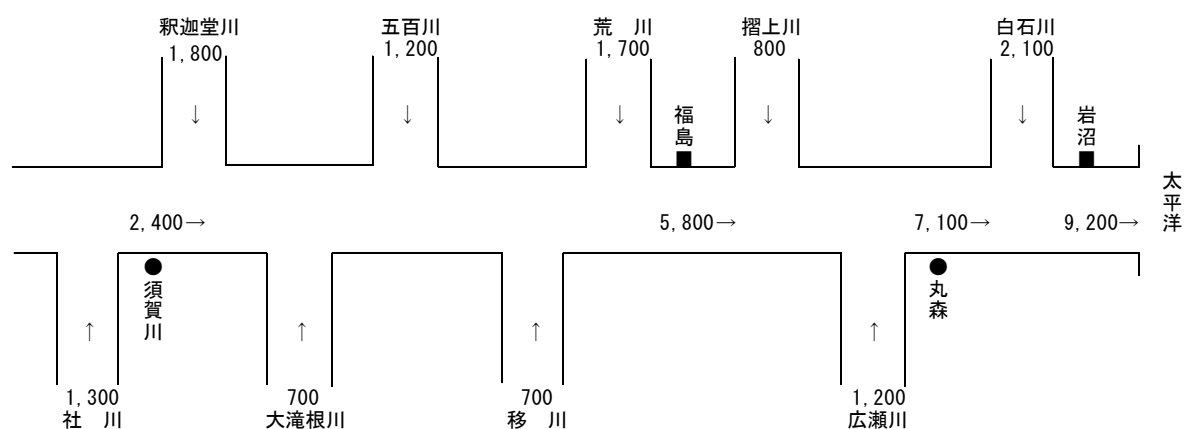
阿武隈川計画高水流量図
