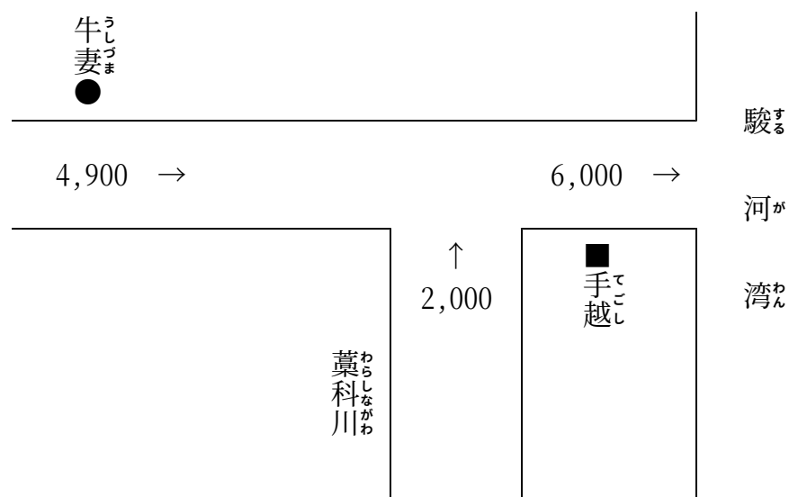
安倍川計画高水流量図（単位： \text{m}^3/\text{s} ）
