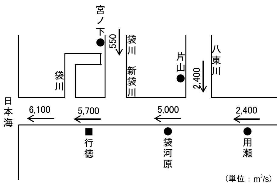
千代川計画高水流量図
