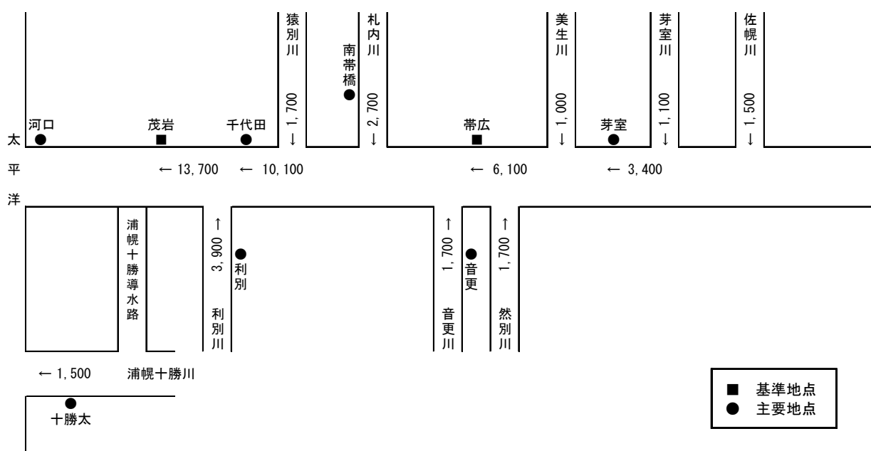
十勝川計画高水流量図
