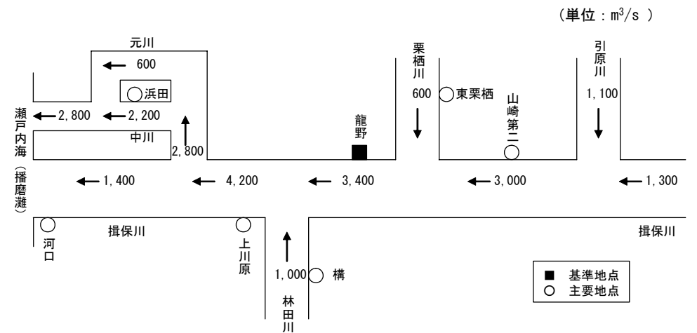
揖保川計画高水流量図
