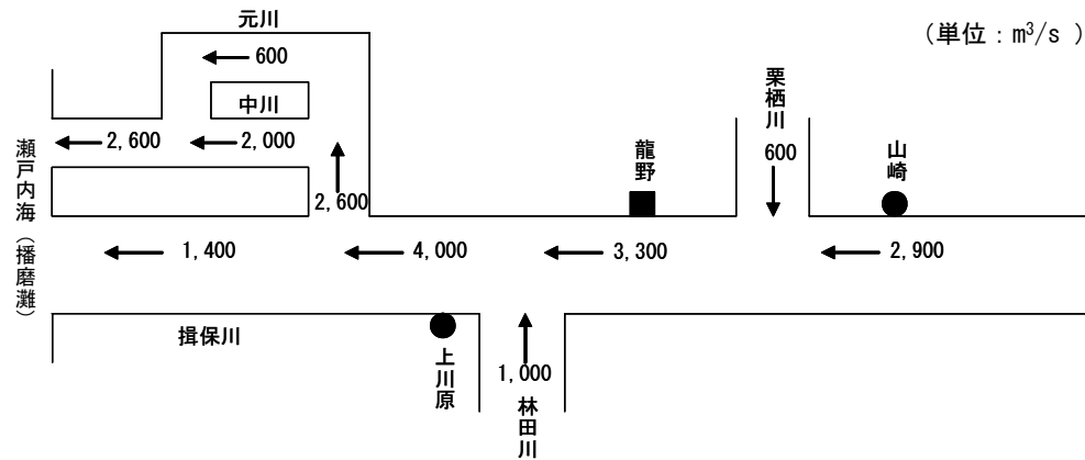
揖保川計画高水流量図
