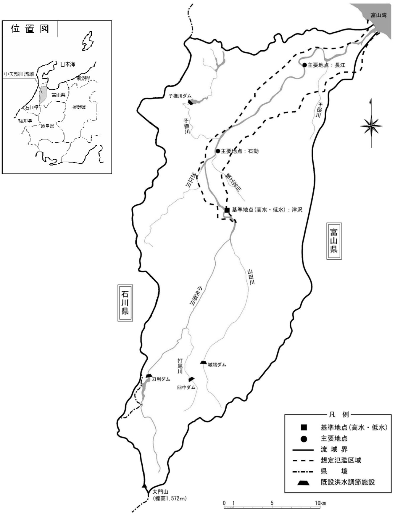
(参考図) 小矢部川水系図
