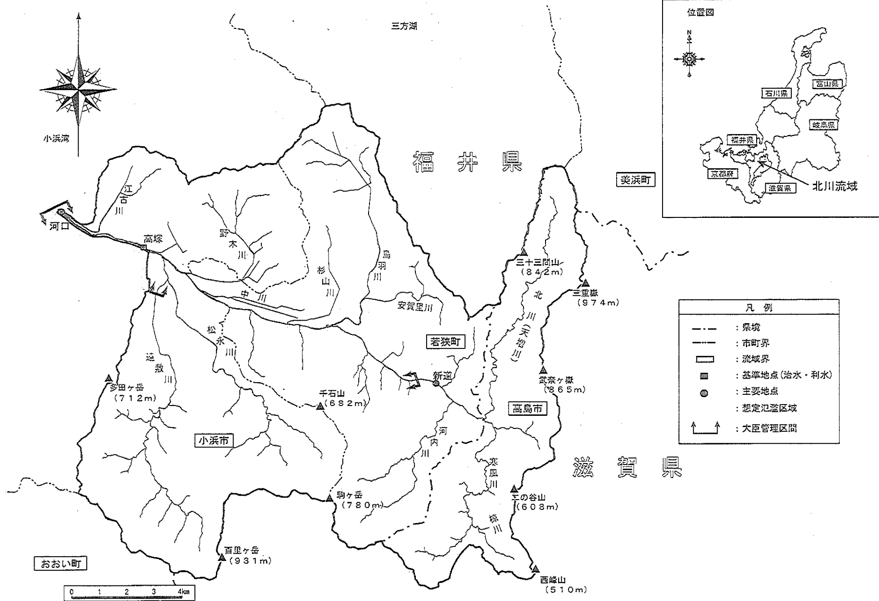
(参考図) 北川水系流域図
