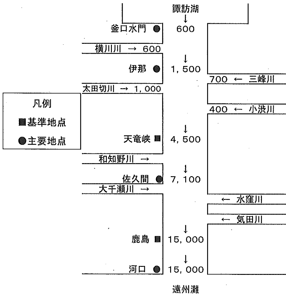
天竜川計画高水流量図 (単位： \text{m}^3/\text{s} )
