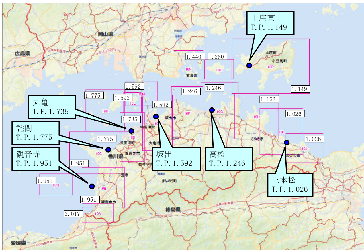
図-7 解析モデルにおける初期潮位の設定範囲図
