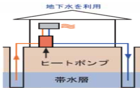
地下水ヒートポンプのイメージ
