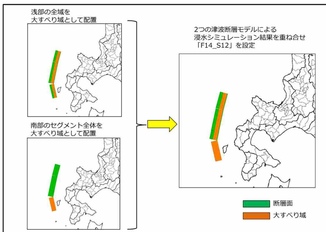
図ー8 津波断層モデル「F14_S12」の考え方
