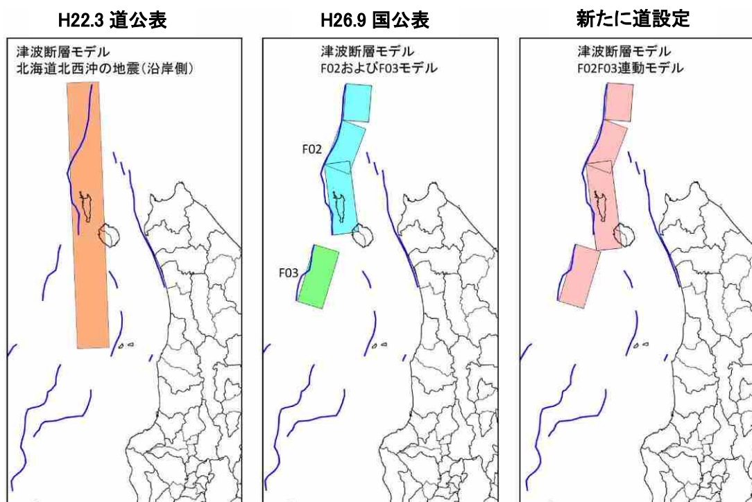
図－10 F02 と F03 を連動した津波断層モデル「F02F03 連動」
