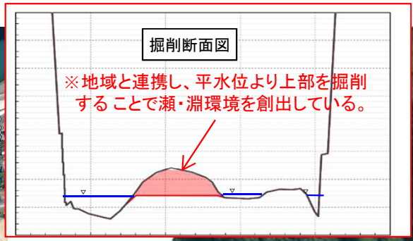
瀬や淵等の環境に配慮した掘削を実施
