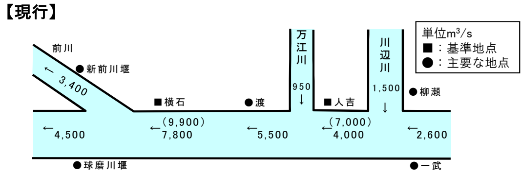
＜球磨川計画高水流量図＞
