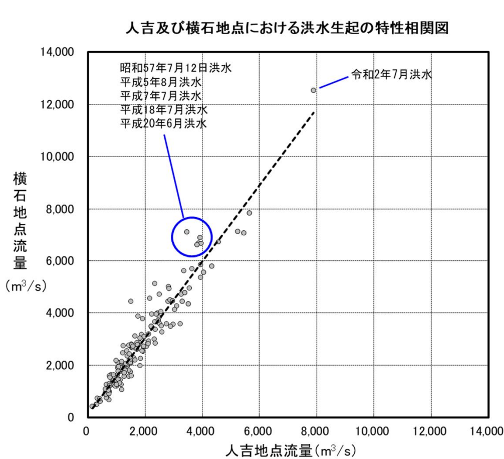
人吉地点と横石地点の洪水流量
