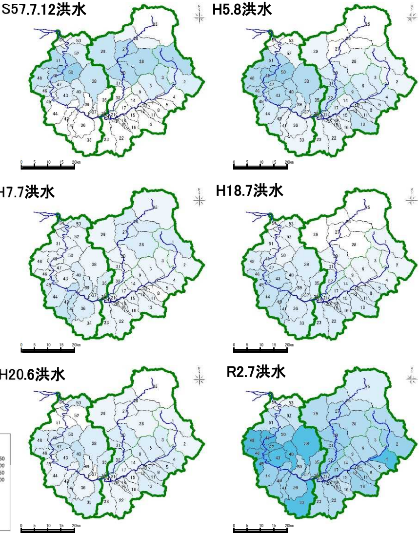
人吉地点と横石地点の流量相関に対し、横石の流量が多い洪水の降雨分布
