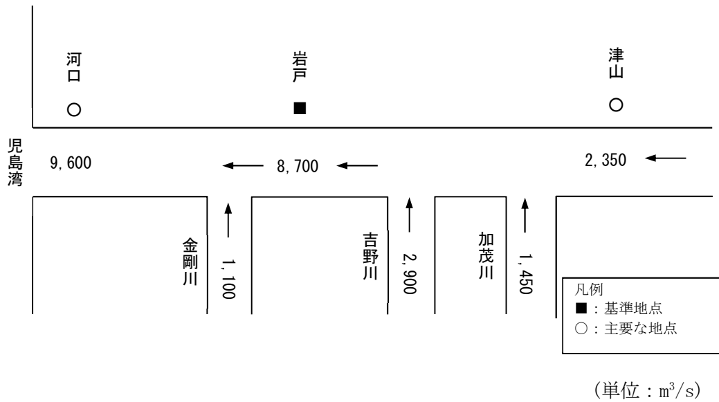
吉井川計画高水流量図
