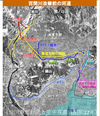
百間川の整備により、治水（岡山城下の浸水被害の軽減）と新田開発（人口増加による食料増産対策）を両立させた
