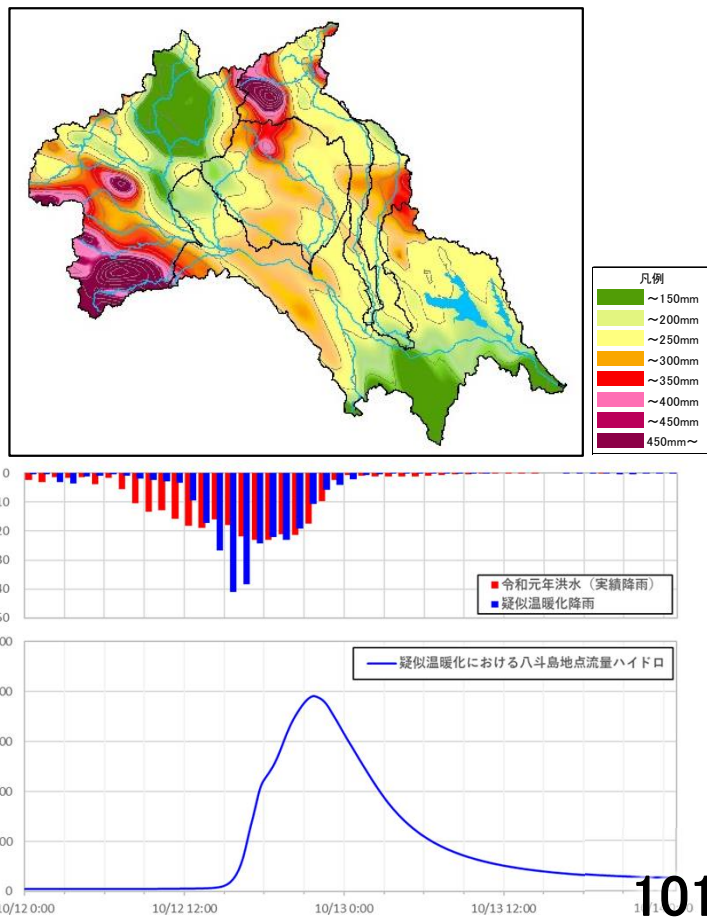
③CReSSモデル(06p)
