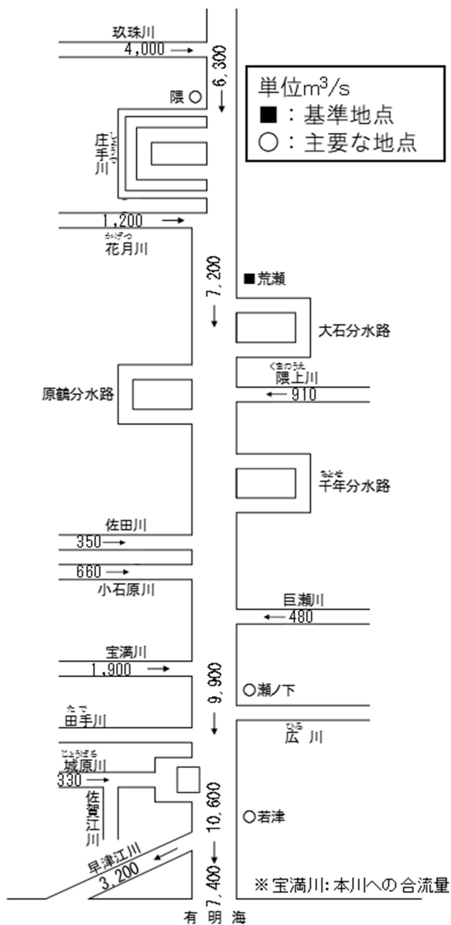
筑後川計画高水流量図
