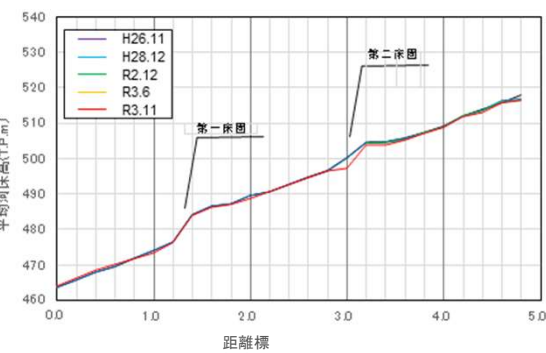
◆平均河床高縦断図(小湫川)
