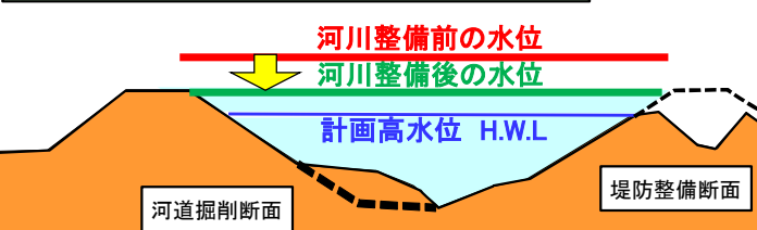
横断面図(支川鍋谷川(梯川合流点上流5km付近))
