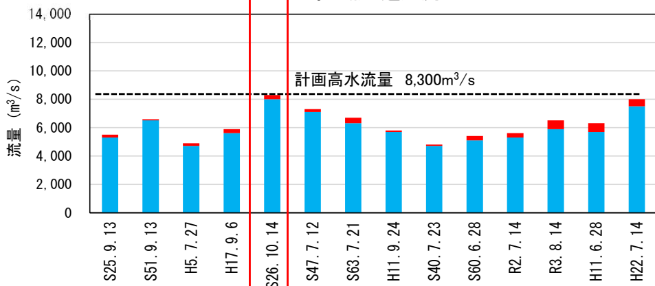
西原地点 通過流量
