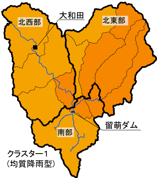
HFB_2K_GF_m108_2073 (12時間雨量) 大和田地点ピーク流量 1,536m 3 /s
