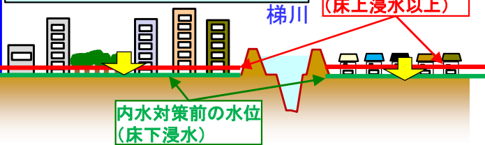
横断面イメージ(梯川及び小松市街地)
