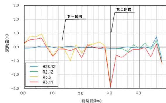
◆平均河床變動量図(小渋川)
