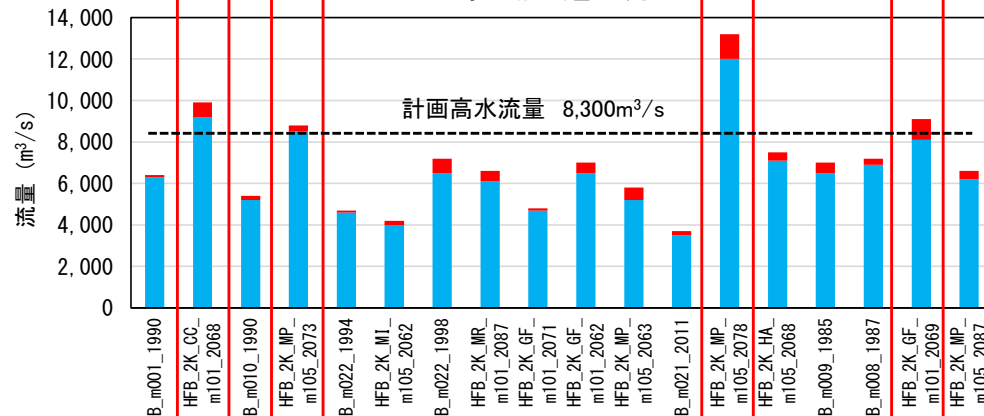
西原地点 通過流量
