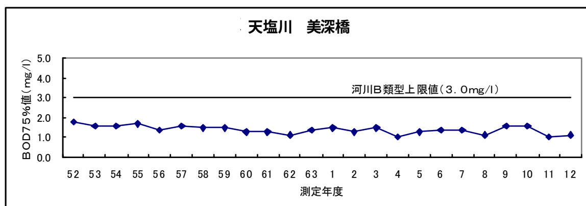
図－2 1 (1) 天塩川の各水質観測地点における BOD75%値の経年変化
