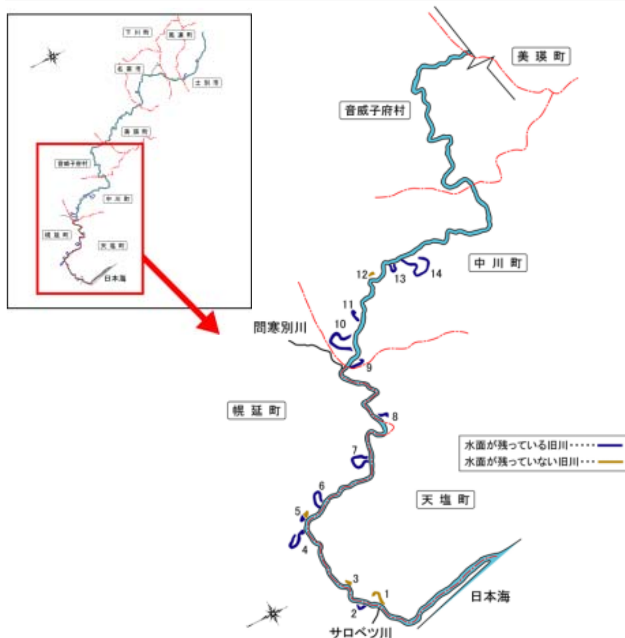
図－８－１ 捷水路工事箇所図
