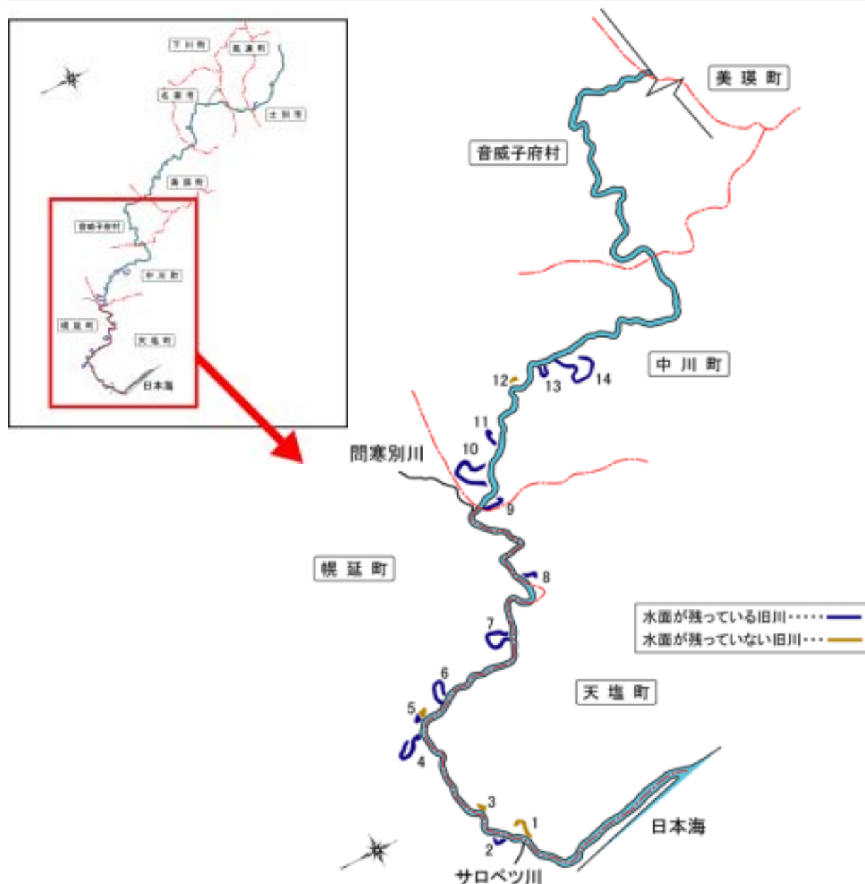
図-8-1 捷水路工事箇所図
