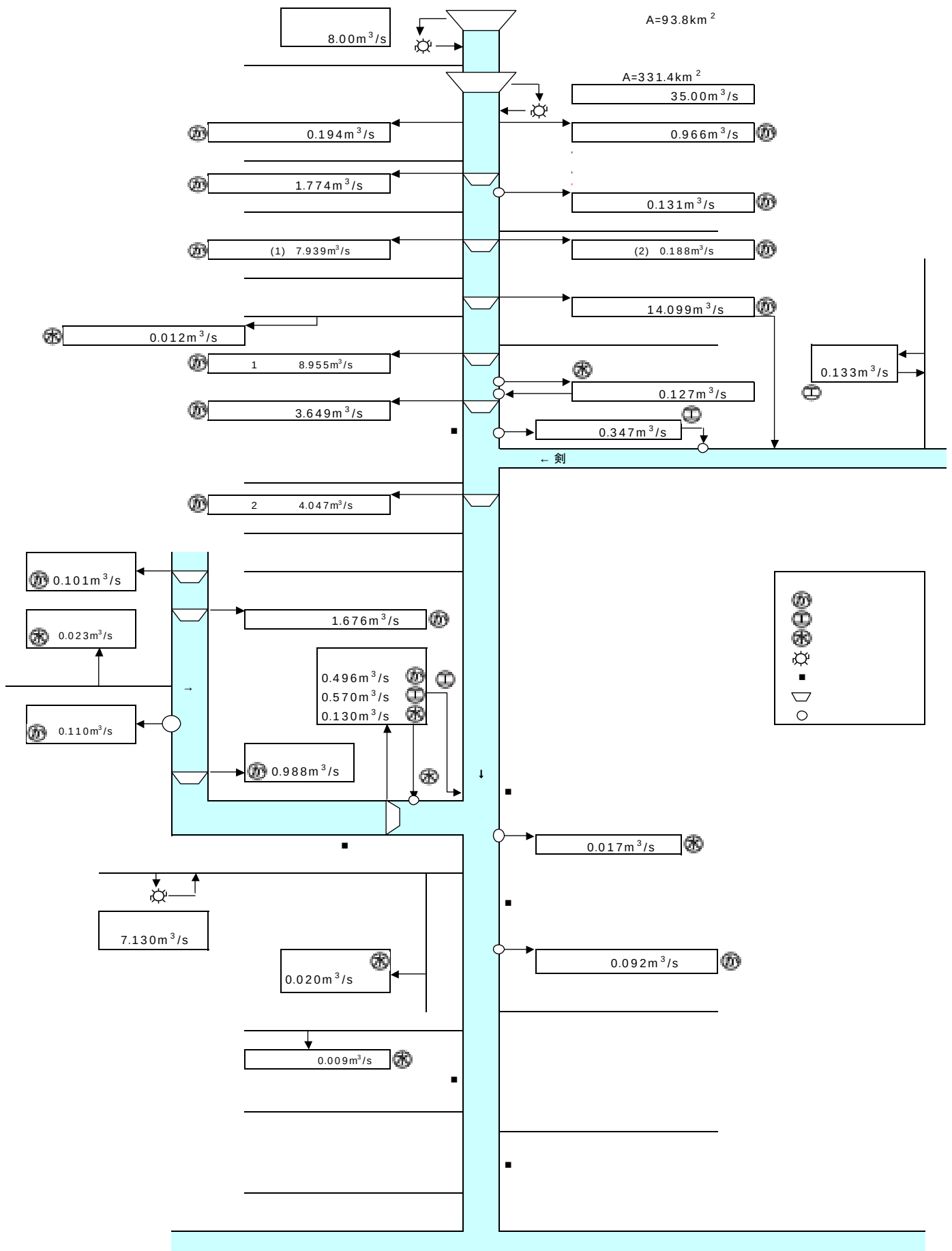
図－１９ 天塩川水系取排水図
