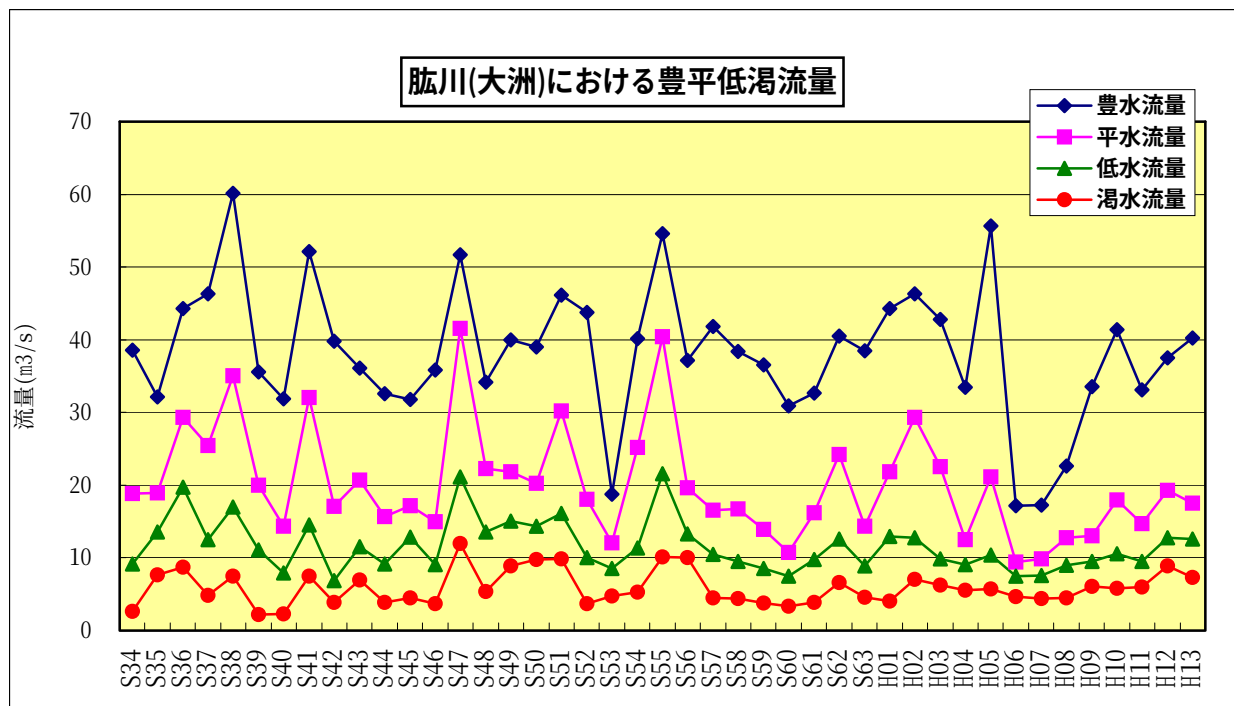
図 6-1 肱川の流況
