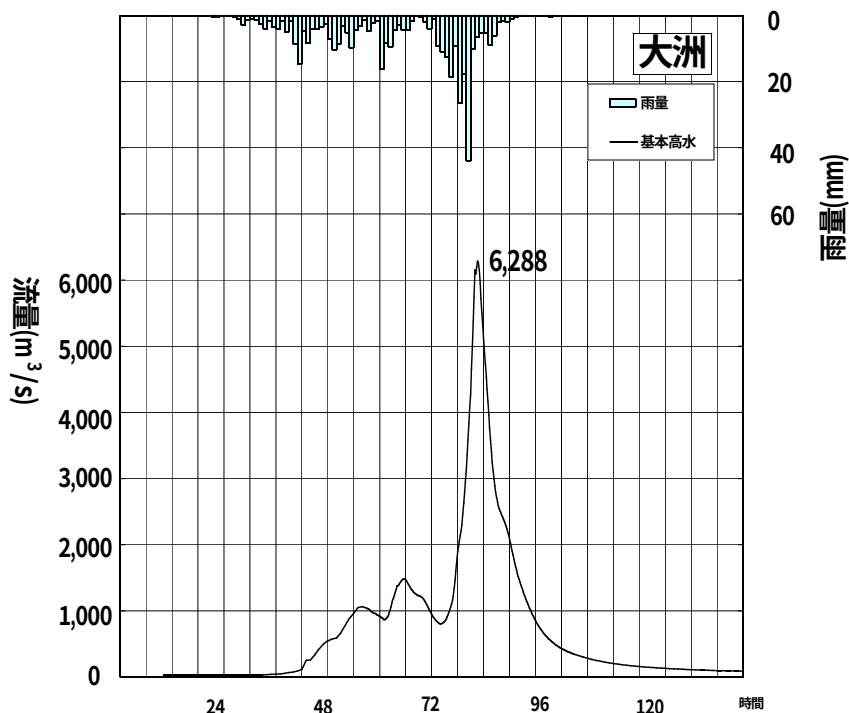
図ー2 基本高水ハイドログラフ (平成2年9月洪水)
