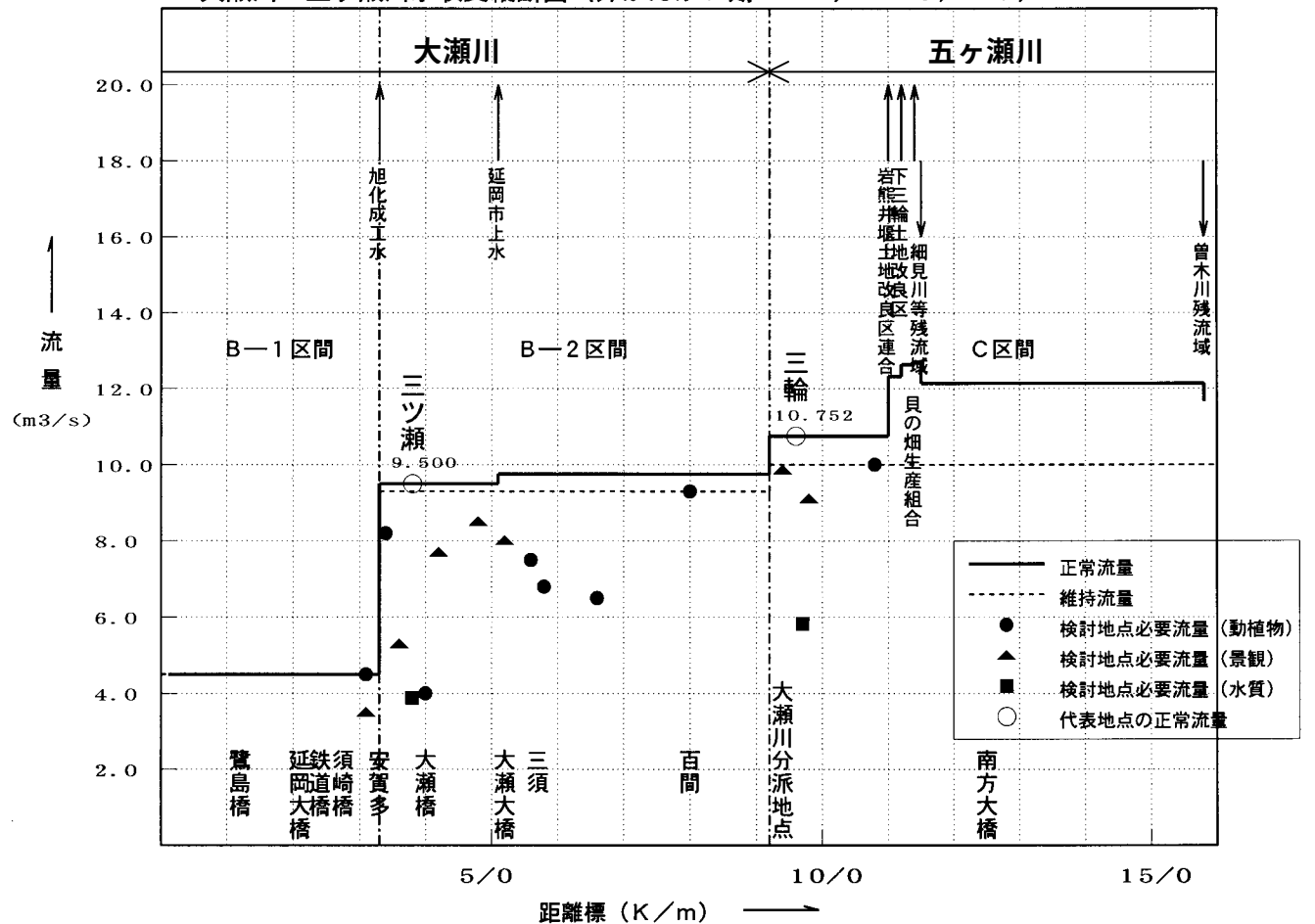
大瀬川・五ヶ瀬川水収支縦断図（非かんがい期1：2／1～6／18）
