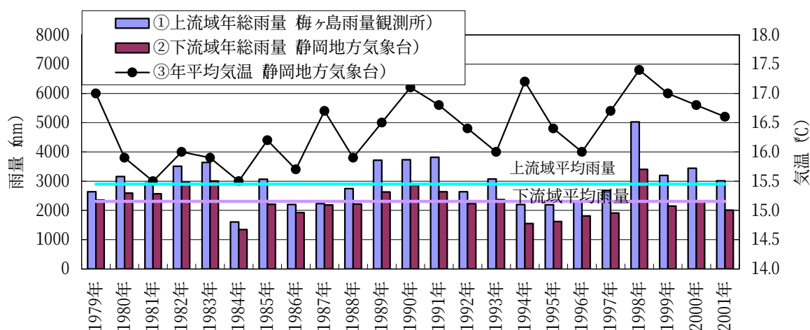
図－1.5 安倍川流域総雨量経年変化図
