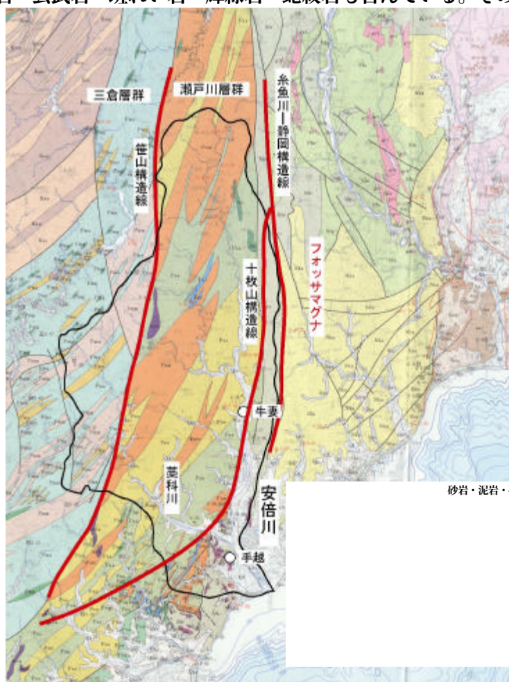
図ー1.4 安倍川流域地質分布図
