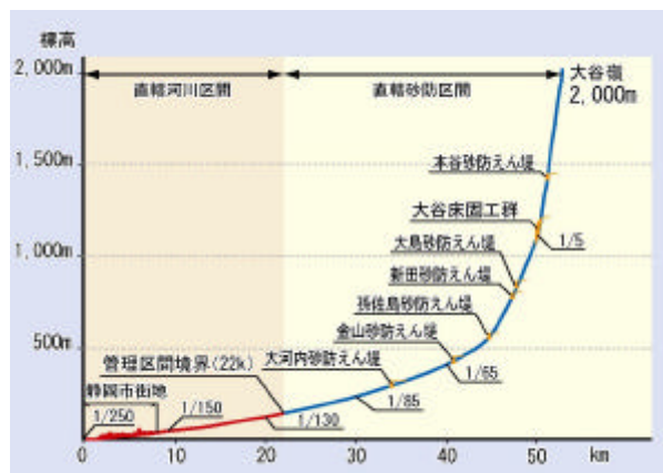
図－8.2 安倍川縦断図
