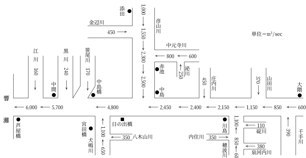
図 4-2 遠賀川現計画高水流量配分図
