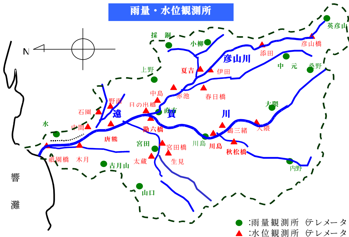
図8-4-1. 雨量・水位観測所位置図
